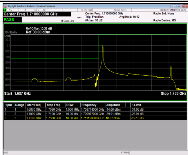
Band4-20MHz-QPSK-20050-100RB#0
