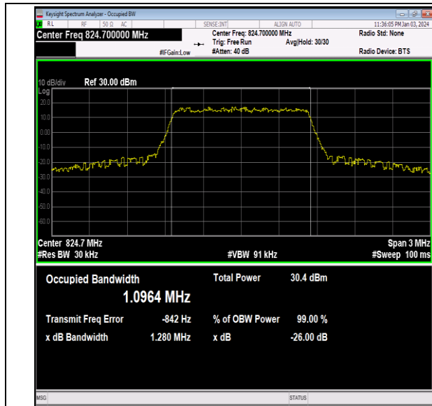
26(824-849)-1.4MHz-QPSK-26797-6RB#0-PASS
