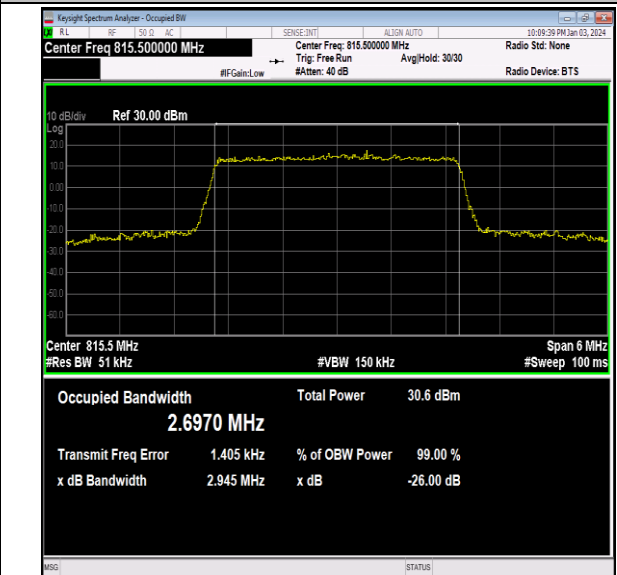
26(814-824)-3MHz-QPSK-26705-15RB#0-PASS
