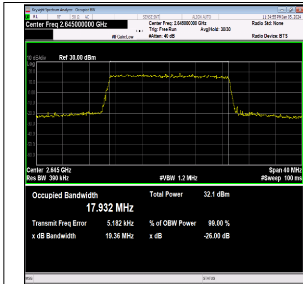
41(2535-2655)-20MHz-QPSK-41140-100RB#0-PASS
