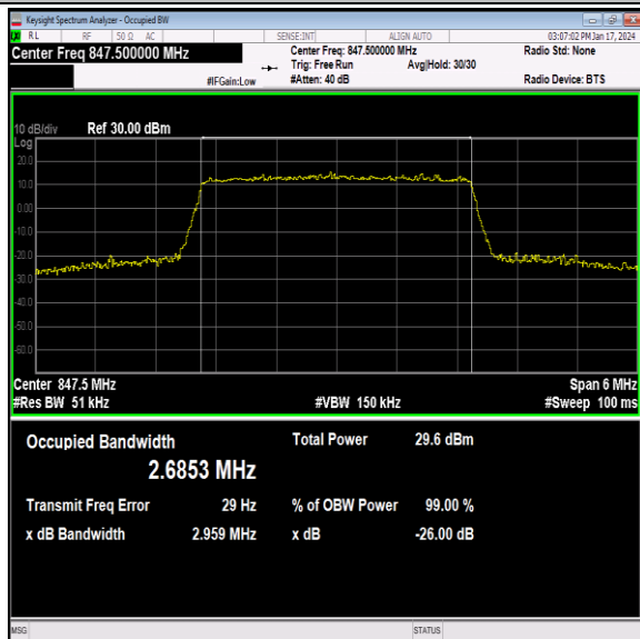
26(824-849)-3MHz-16QAM-27025-15RB#0-PASS
