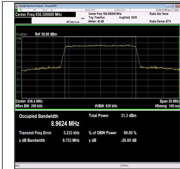
26(824-849)-10MHz-QPSK-26915-50RB#0-PASS
