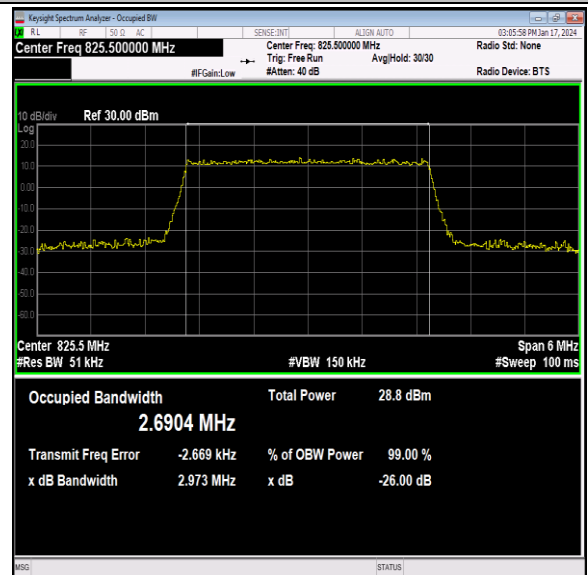
26(824-849)-3MHz-64QAM-26805-15RB#0-PASS
