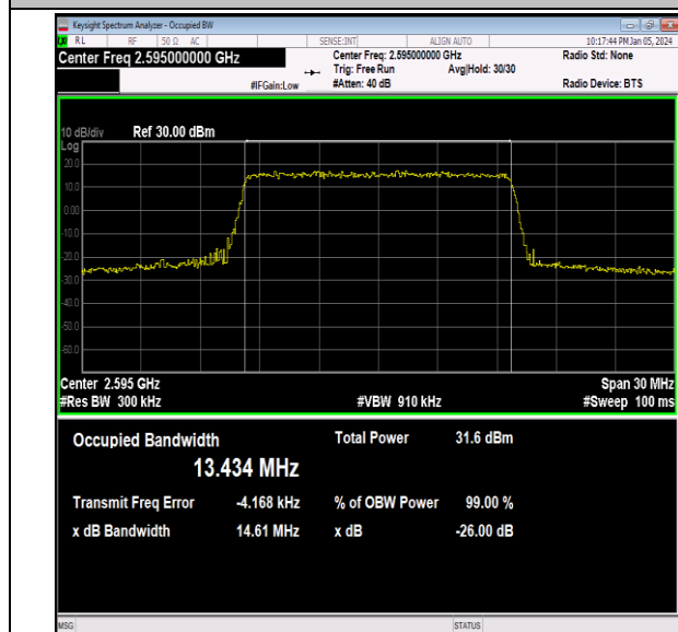
41(2535-2655)-15MHz-QPSK-40640-75RB#0-PASS
