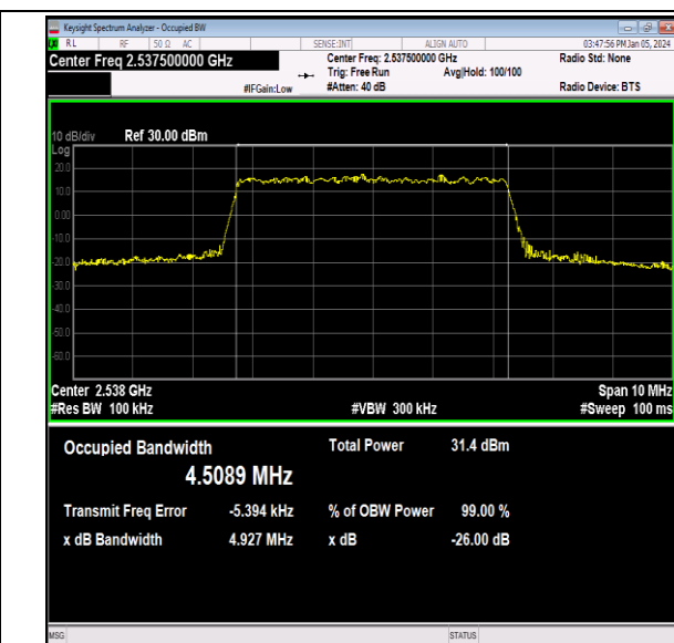
41(2535-2655)-5MHz-QPSK-40065-25RB#0-PASS
