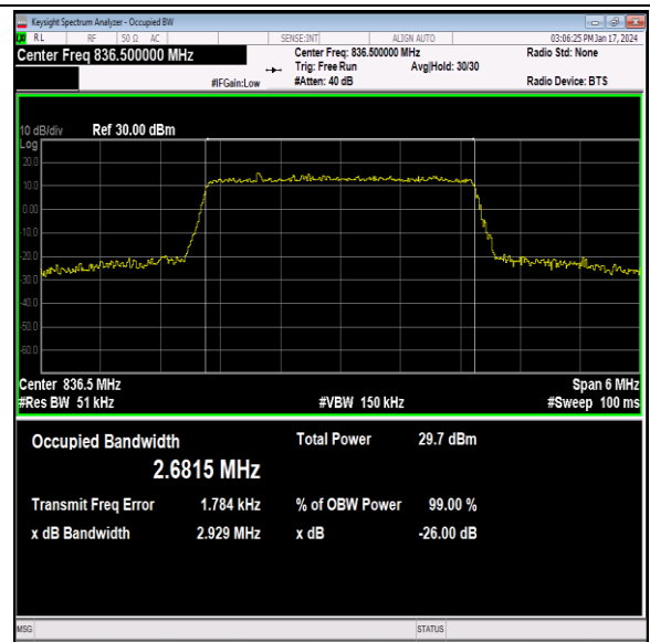
26(824-849)-3MHz-16QAM-26915-15RB#0-PASS
