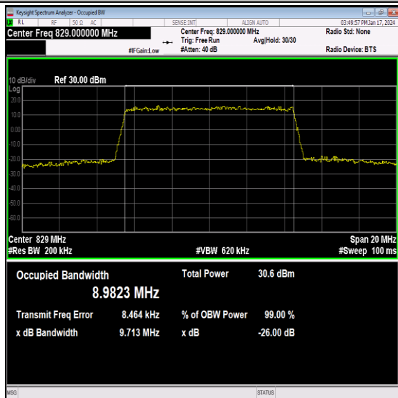
26(824-849)-10MHz-16QAM-26840-50RB#0-PASS
