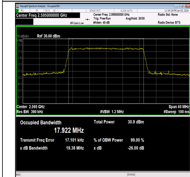
41(2535-2655)-20MHz-16QAM-40640-100RB#0-PASS
