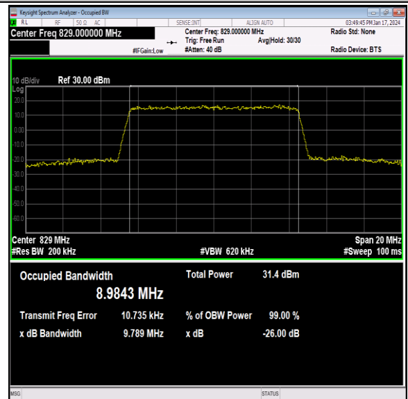
26(824-849)-10MHz-QPSK-26840-50RB#0-PASS
