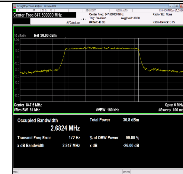
26(824-849)-3MHz-QPSK-27025-15RB#0-PASS
