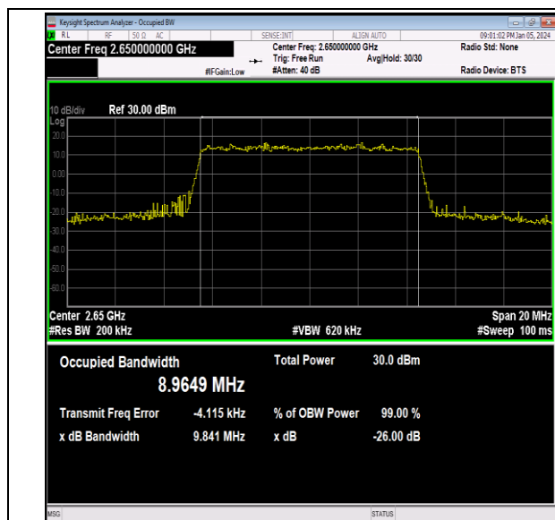
41(2535-2655)-10MHz-64QAM-41190-50RB#0-PASS
