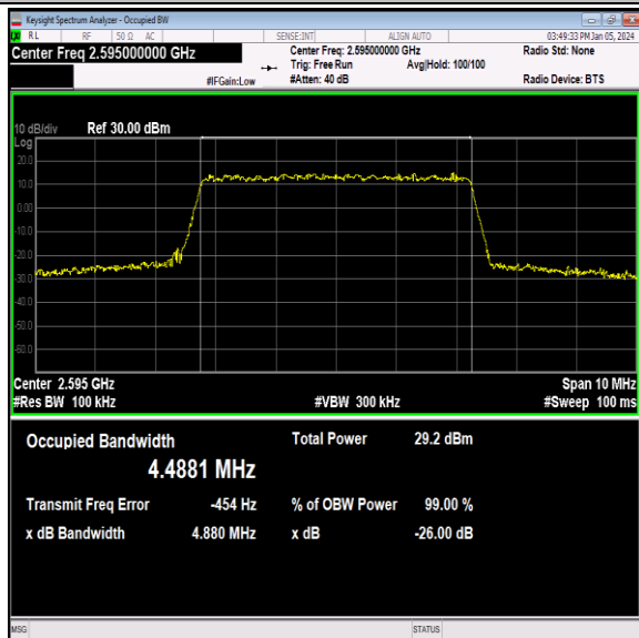
41(2535-2655)-5MHz-64QAM-40640-25RB#0-PASS
