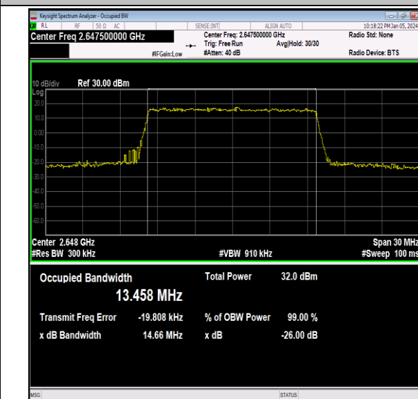
41(2535-2655)-15MHz-QPSK-41165-75RB#0-PASS
