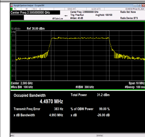
41(2535-2655)-5MHz-QPSK-40640-25RB#0-PASS
