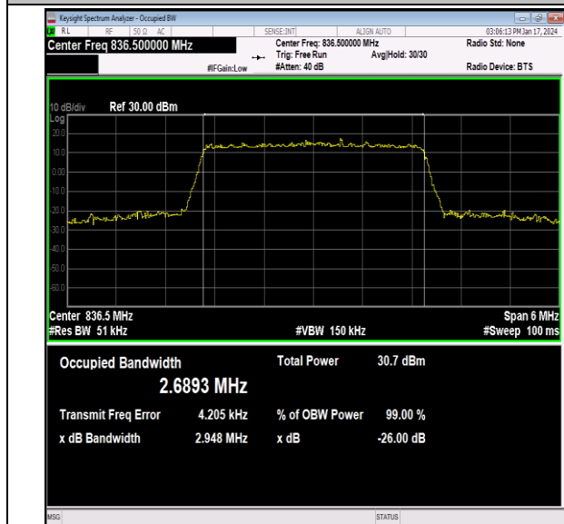
26(824-849)-3MHz-QPSK-26915-15RB#0-PASS
