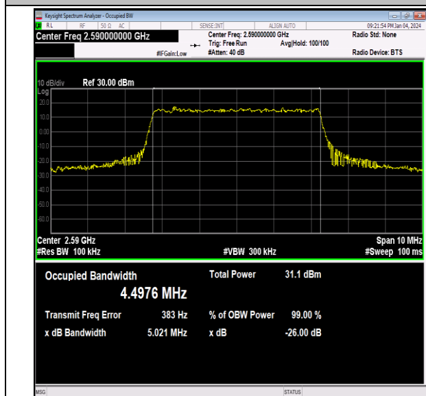
41(2535-2655)-5MHz-QPSK-40590-25RB#0-PASS
