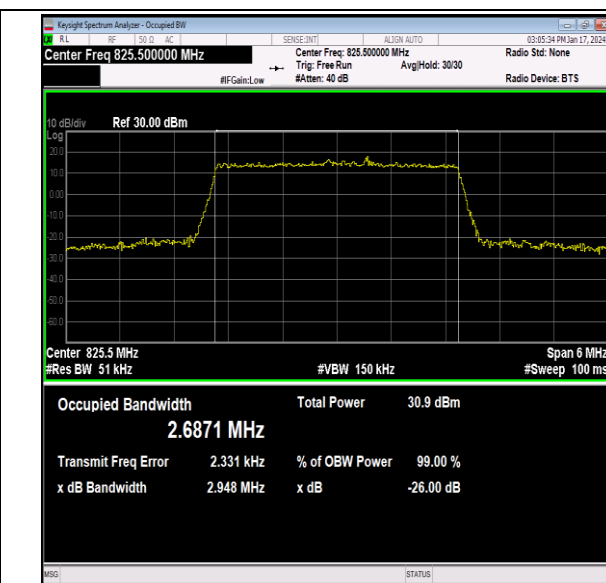
26(824-849)-3MHz-QPSK-26805-15RB#0-PASS
