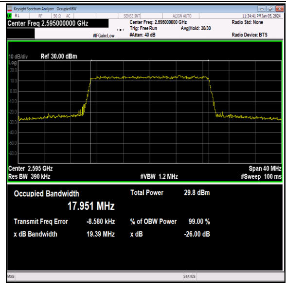
41(2535-2655)-20MHz-64QAM-40640-100RB#0-PASS
