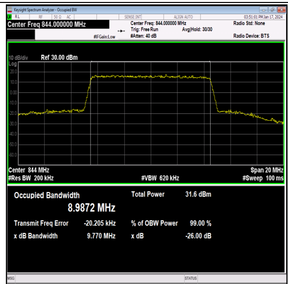
26(824-849)-10MHz-QPSK-26990-50RB#0-PASS
