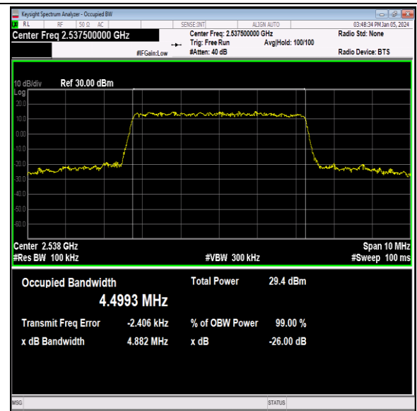
41(2535-2655)-5MHz-64QAM-40065-25RB#0-PASS
