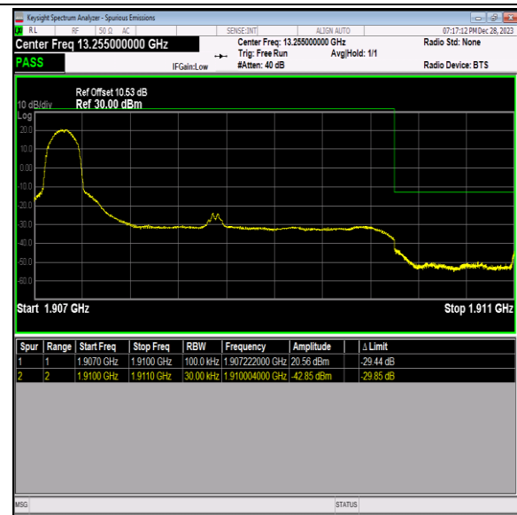
Band2_3MHz_QPSK_19185_1RB#0
