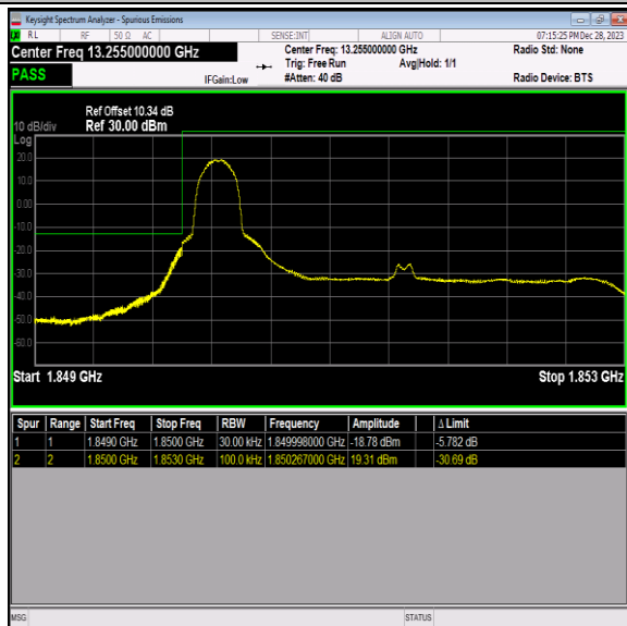
Band2_3MHz_QPSK_18615_1RB#0
