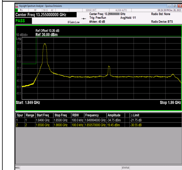
Band2_10MHz_QPSK_18650_1RB#0
