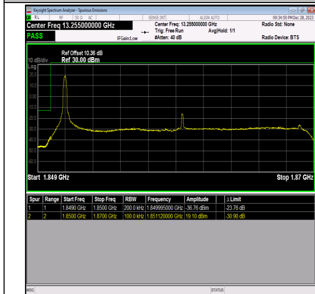
Band2_20MHz_QPSK_18700_1RB#0
