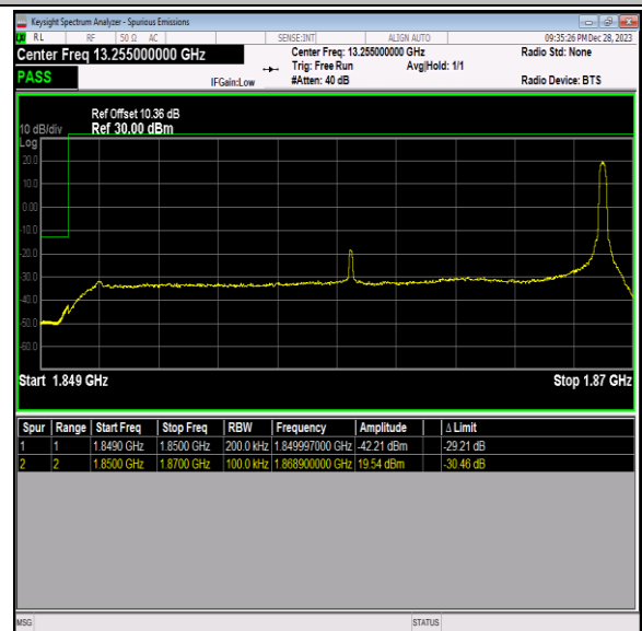
Band2_20MHz_QPSK_18700_1RB#99
