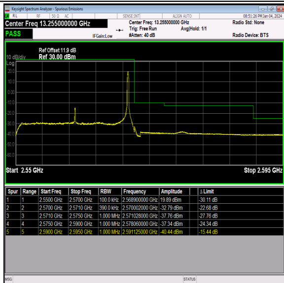
Band7_20MHz_QPSK_21350_1RB#99
