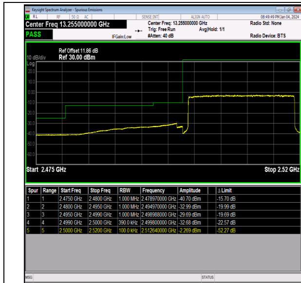
Band7_20MHz_QPSK_20850_100RB#0
