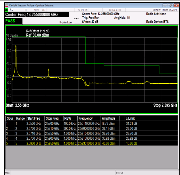
Band7_20MHz_16QAM_21350_1RB#0
