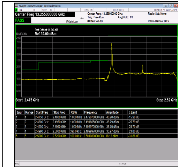
Band7_20MHz_16QAM_20850_1RB#0
