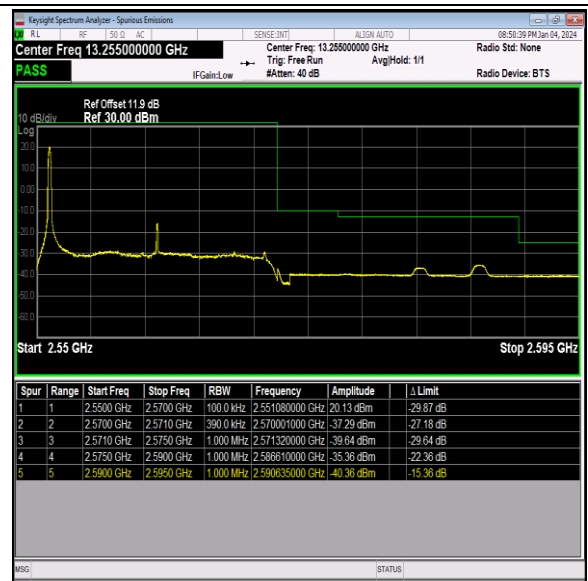
Band7_20MHz_QPSK_21350_1RB#0
