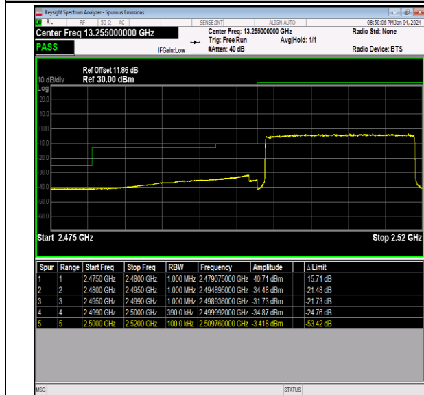
Band7_20MHz_16QAM_20850_100RB#0
