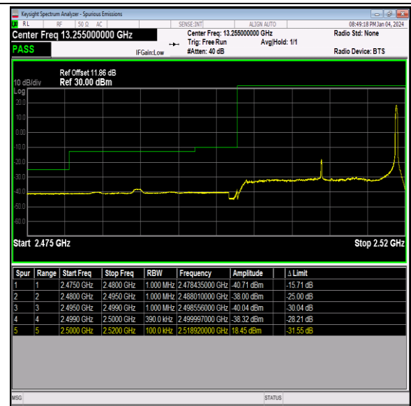
Band7_20MHz_16QAM_20850_1RB#99
