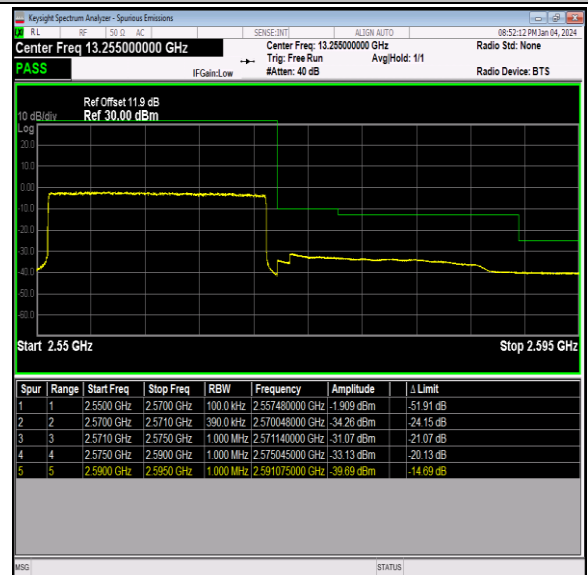
Band7_20MHz_QPSK_21350_100RB#0
