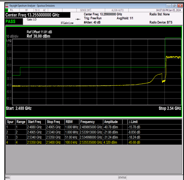
Band41_5MHz_QPSK_40065_25RB#0
