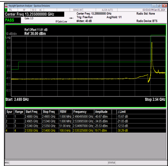
Band41_5MHz_QPSK_40065_1RB#0
