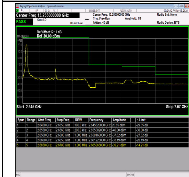
Band41_10MHz_QPSK_41190_1RB#0
