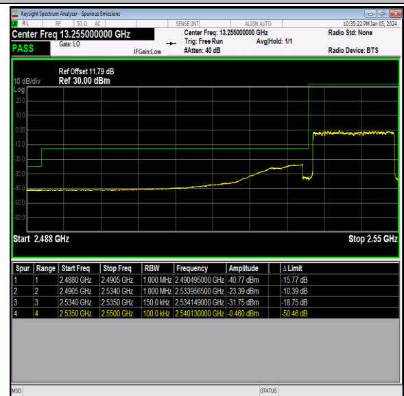
Band41_15MHz_QPSK_40115_75RB#0
