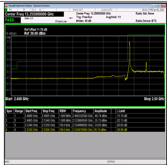
Band41_15MHz_QPSK_40115_1RB#0
