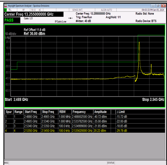
Band41_10MHz_QPSK_40090_1RB#0
