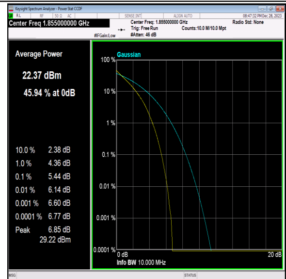
Band2-10MHz-QPSK-18650-50RB#0-PASS
