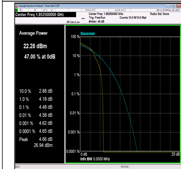
Band2-5MHz-16QAM-18625-1RB#0-PASS
