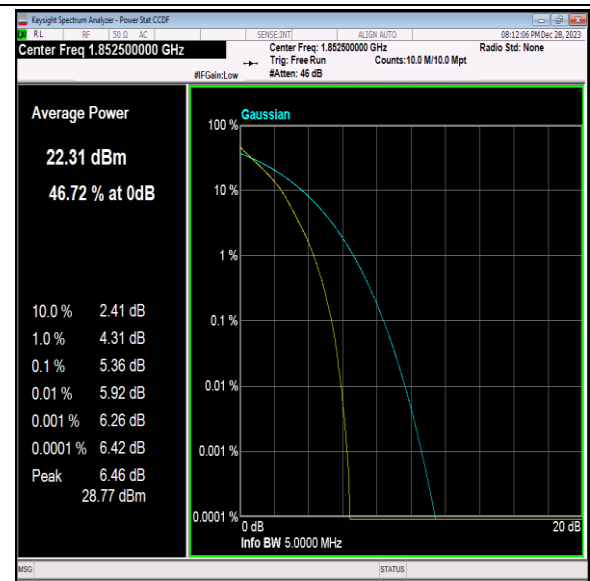
Band2-5MHz-QPSK-18625-25RB#0-PASS
