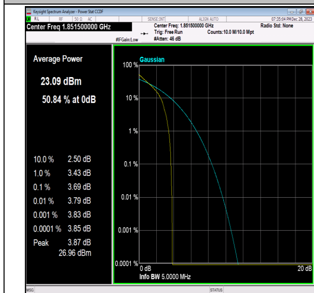
Band2-3MHz-QPSK-18615-1RB#0-PASS
