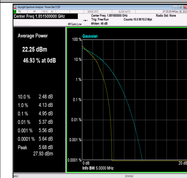
Band2-3MHz-QPSK-18615-15RB#0-PASS
