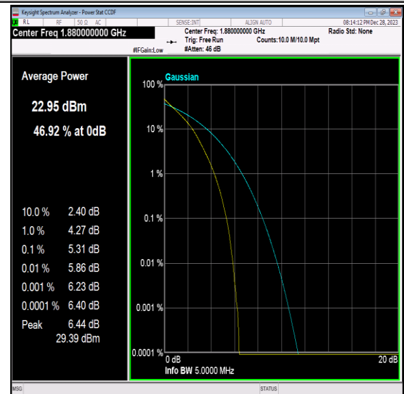
Band2-5MHz-QPSK-18900-25RB#0-PASS
