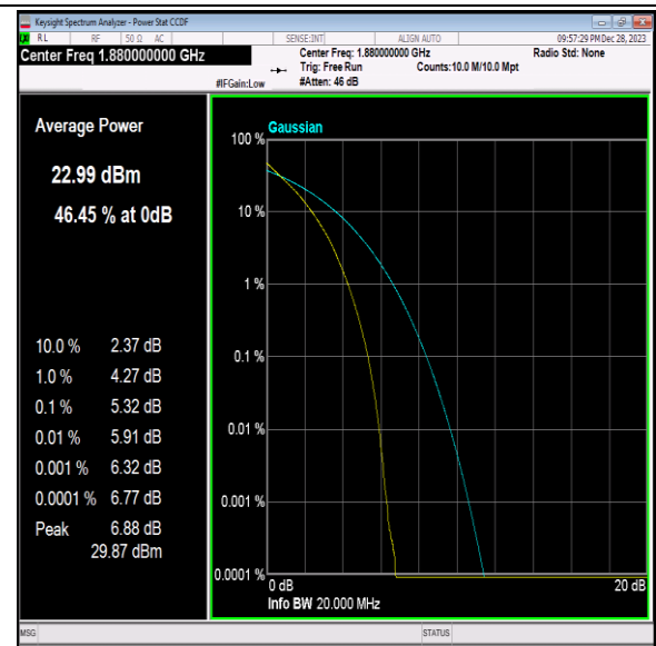
Band2-20MHz-QPSK-18900-100RB#0-PASS
