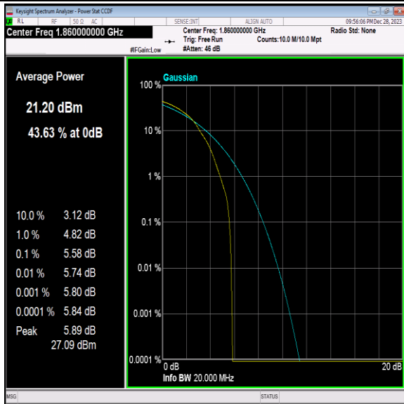
Band2-20MHz-64QAM-18700-1RB#0-PASS
