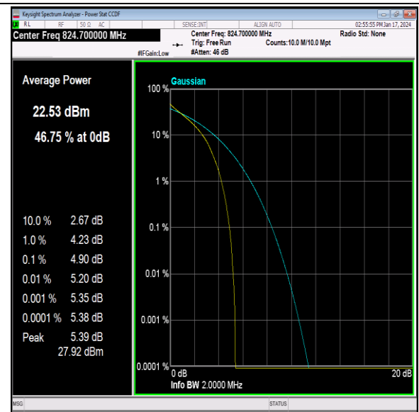
26(824-849)-1.4MHz-QPSK-26797-6RB#0-PASS
