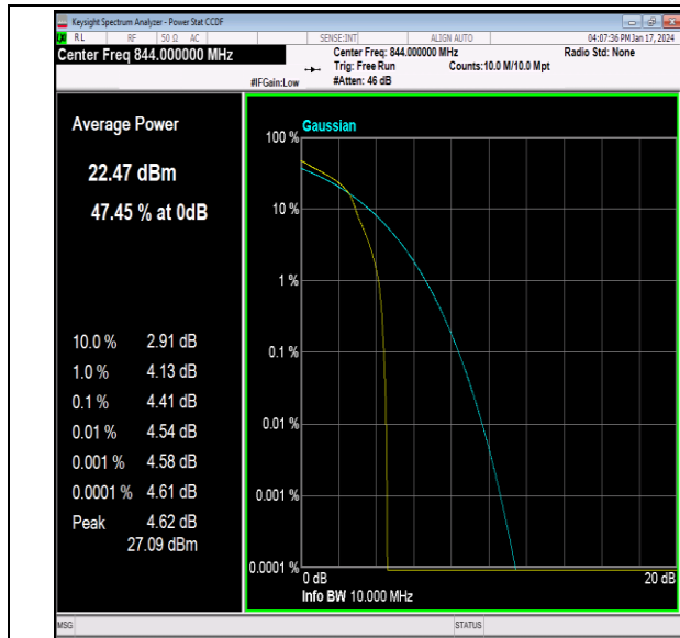
26(824-849)-10MHz-16QAM-26990-1RB#0-PASS
