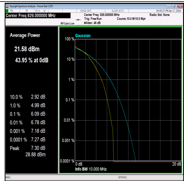
26(824-849)-10MHz-16QAM-26840-50RB#0-PASS
