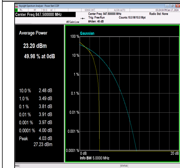
26(824-849)-3MHz-QPSK-27025-1RB#0-PASS
