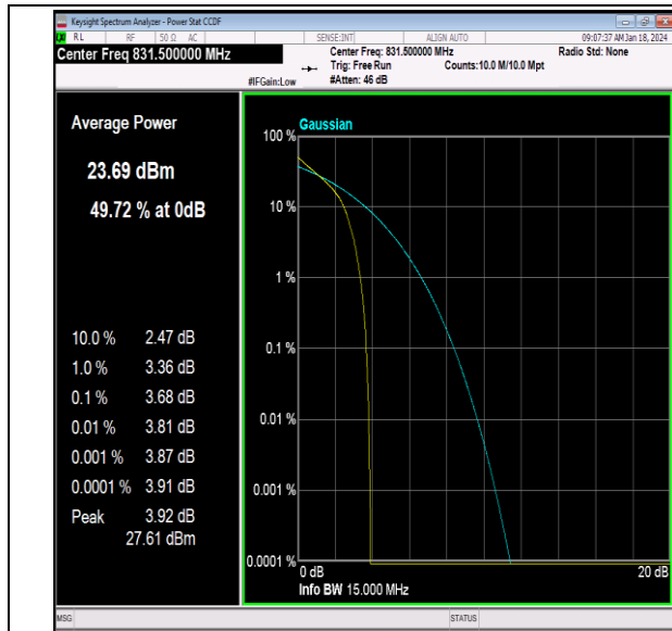
26(824-849)-15MHz-QPSK-26865-1RB#0-PASS
