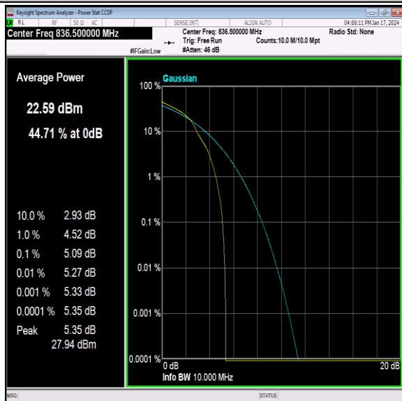
26(824-849)-10MHz-16QAM-26915-1RB#0-PASS
