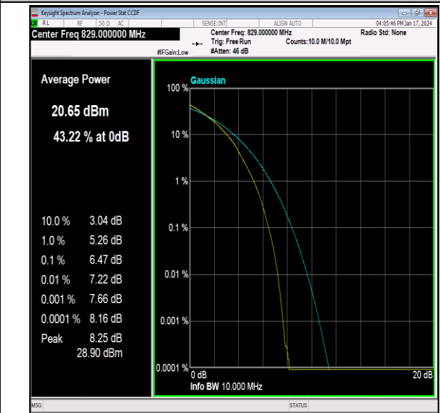
26(824-849)-10MHz-64QAM-26840-50RB#0-PASS
