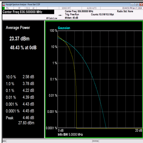
26(824-849)-5MHz-QPSK-26915-1RB#0-PASS
