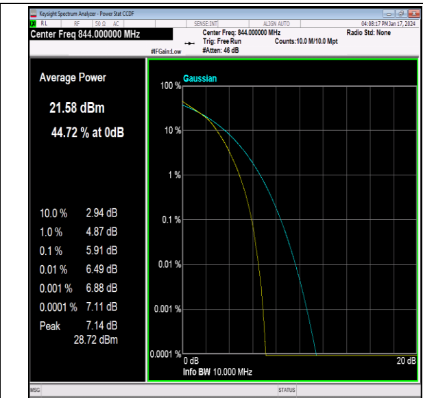
26(824-849)-10MHz-16QAM-26990-50RB#0-PASS
