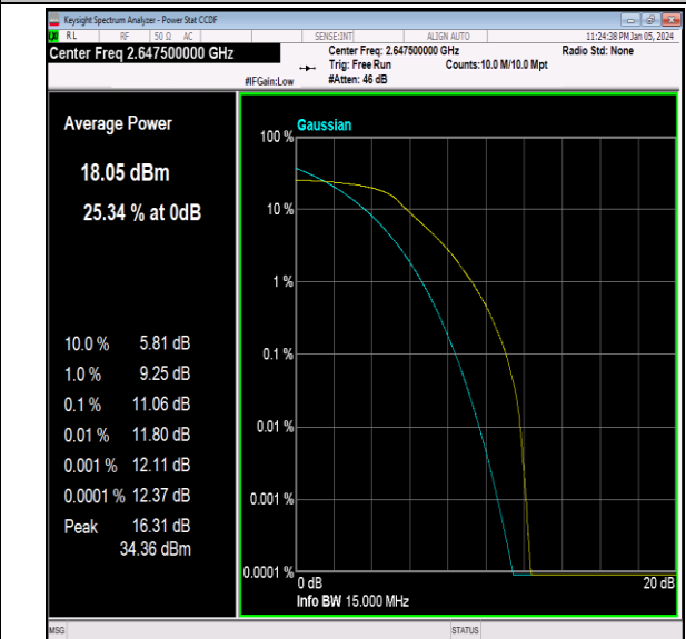
41(2535-2655)-15MHz-QPSK-41165-75RB#0-PASS
