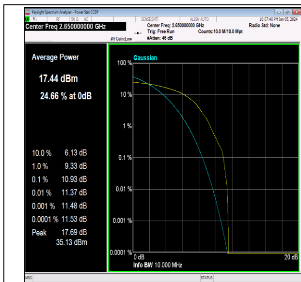
41(2535-2655)-10MHz-64QAM-41190-1RB#0-PASS
