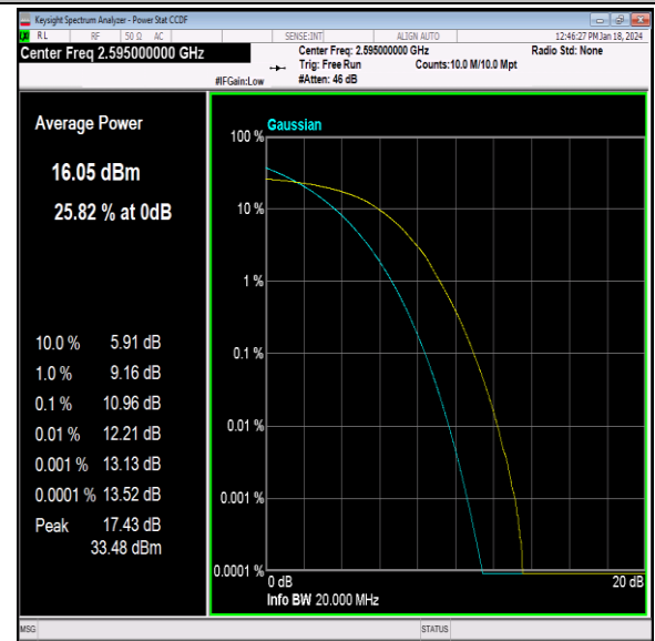
41(2535-2655)-20MHz-64QAM-40640-100RB#0-PASS
