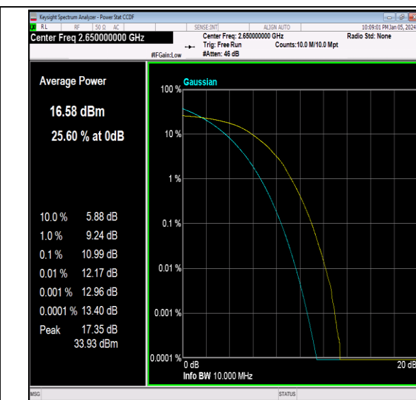
41(2535-2655)-10MHz-64QAM-41190-50RB#0-PASS
