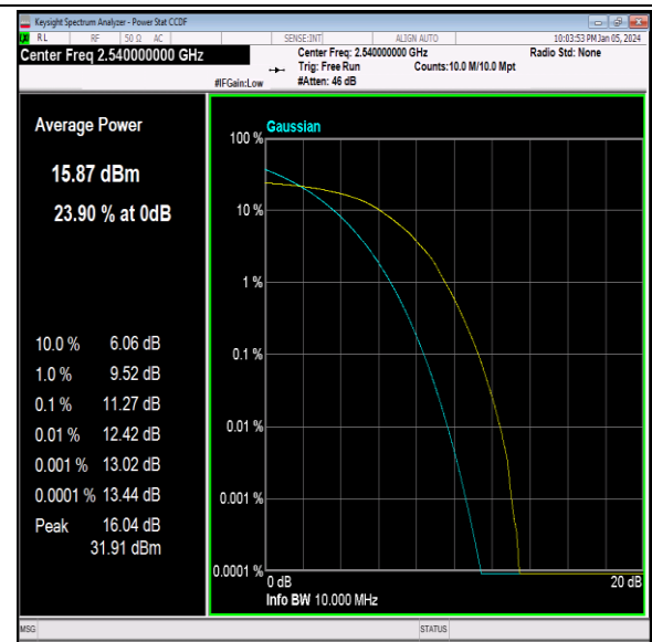
41(2535-2655)-10MHz-64QAM-40090-50RB#0-PASS
