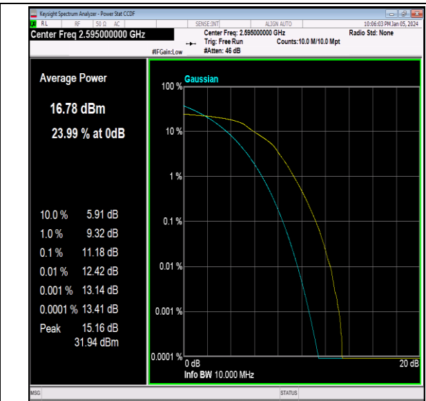
41(2535-2655)-10MHz-16QAM-40640-50RB#0-PASS
