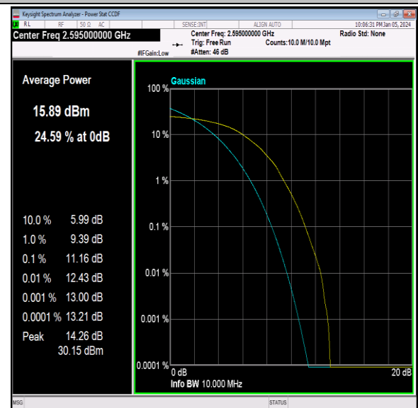
41(2535-2655)-10MHz-64QAM-40640-50RB#0-PASS
