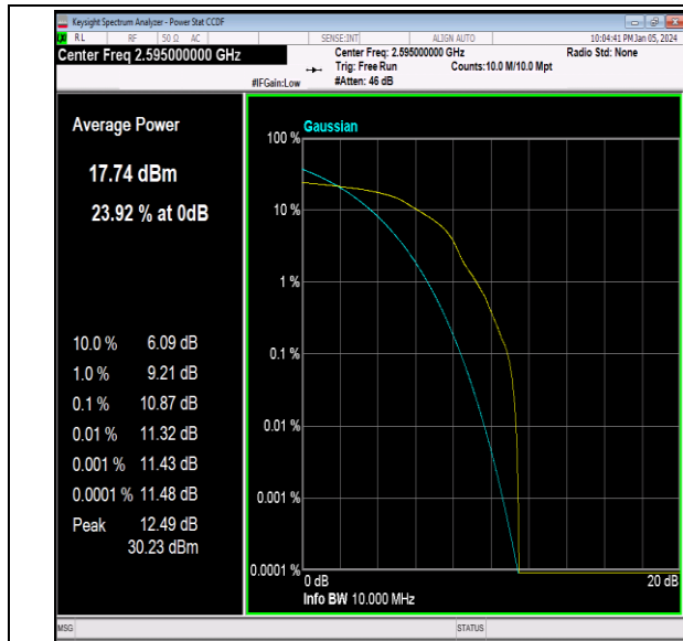
41(2535-2655)-10MHz-16QAM-40640-1RB#0-PASS
