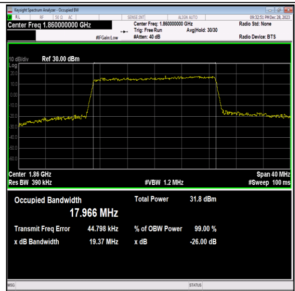
Band2-20MHz-QPSK-18700-100RB#0-PASS
