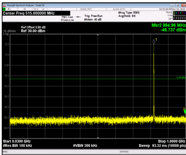
Band26-1.4MHz-QPSK-26797-1RB#0-Range1:30~1 000MHz
