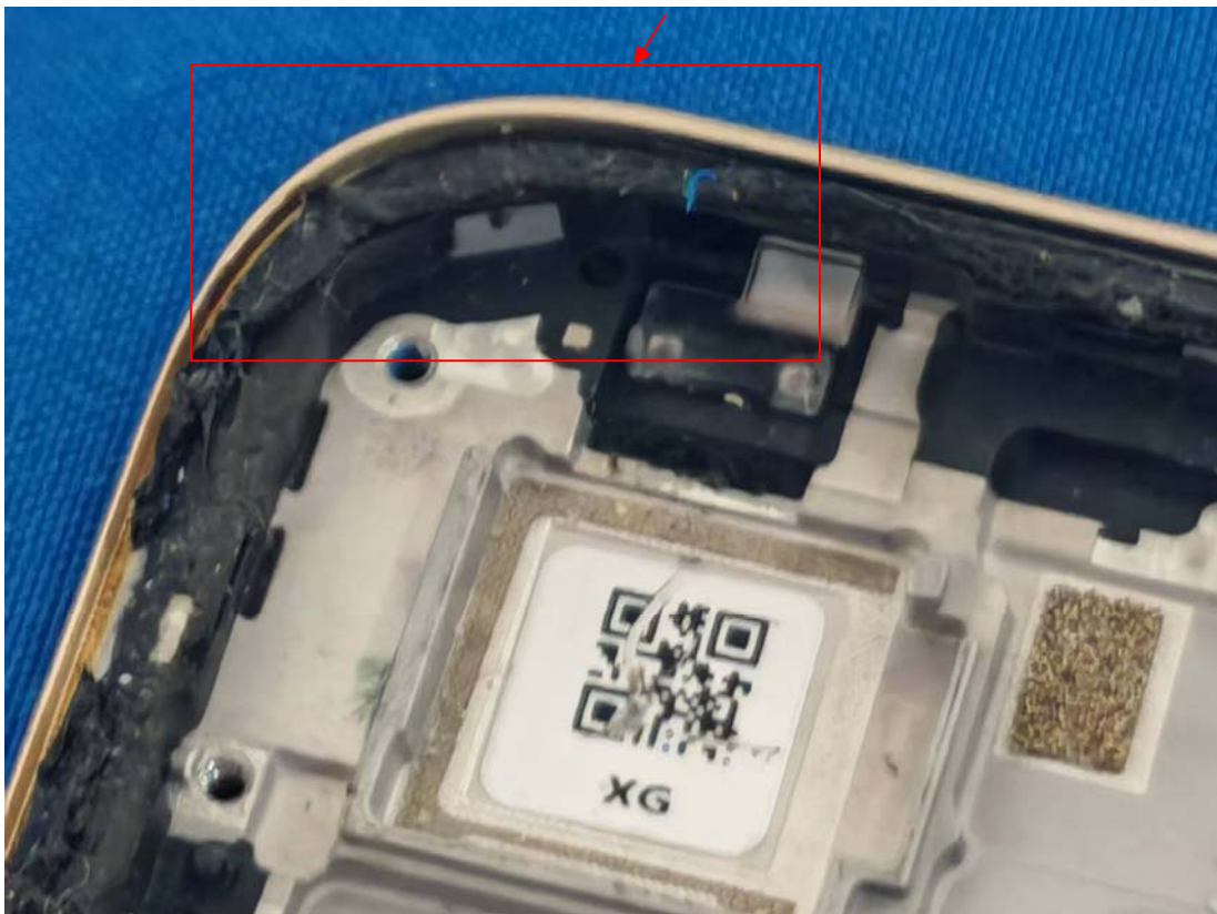
GPS Antenna(ANT 12)
