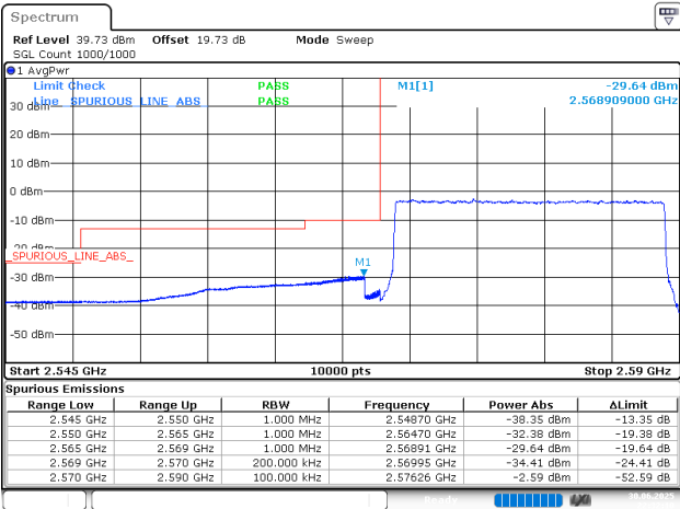
20MHz_Low_QPSK_100@0
