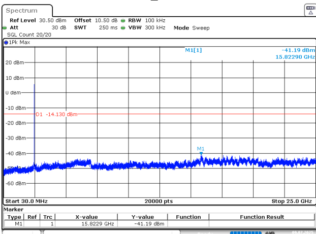
802.11b_2462MHz
