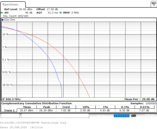
5MHz_Middle_QPSK_25@0
