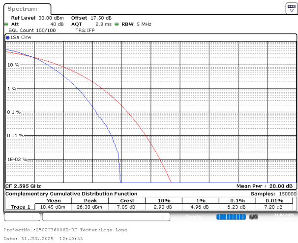
5MHz_Middle_16QAM_25@0
