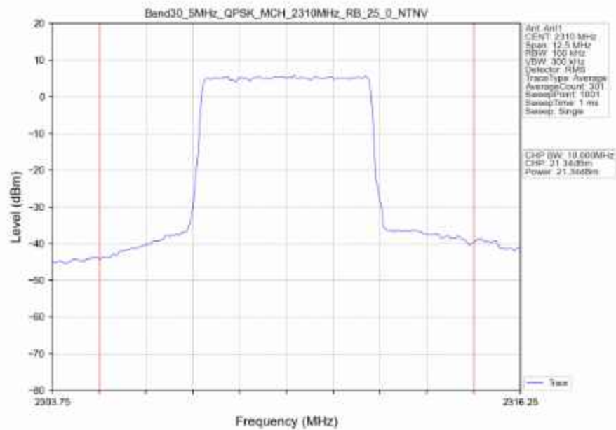
Band30_5MHz_QPSK_MCH_2310MHz_RB_25_0_NTNV
