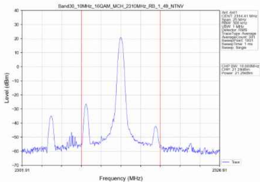
Band30_10MHz_16QAM_MCH_2310MHz_RB_1_49_NTNV
