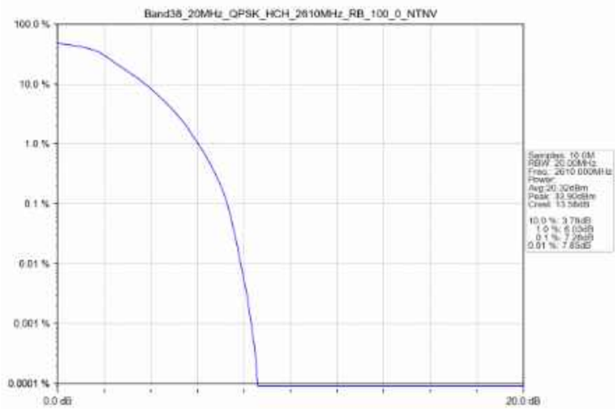
Band38_20MHz_QPSK_HCH_2610MHz_RB_100_0_NTNV
