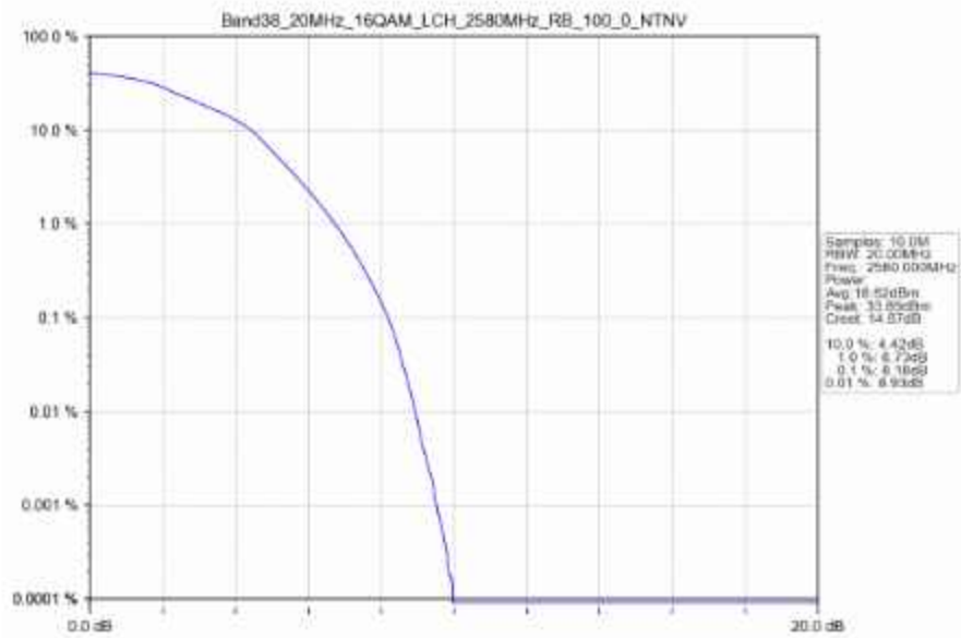
Band38_20MHz_16QAM_LCH_2580MHz_RB_100_0_NTNV
