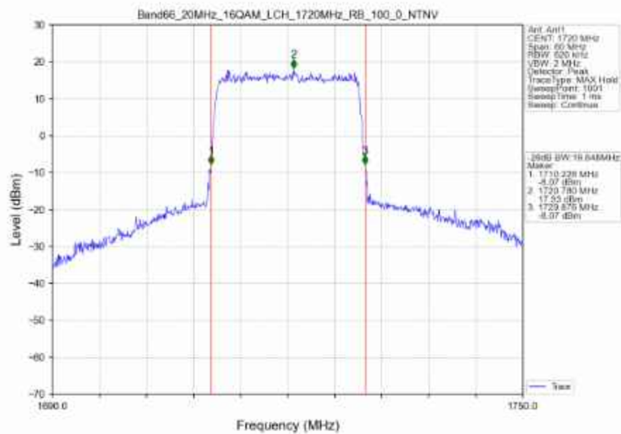
Band66_20MHz_16QAM_LCH_1720MHz_RB_100_0_NTNV
