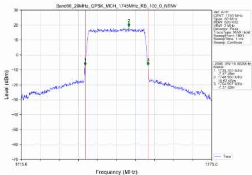
Band66_20MHz_QPSK_MCH_1745MHz_RB_100_0_NTNV
