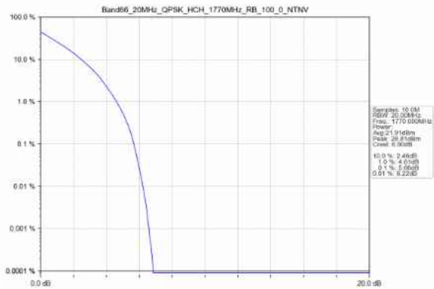
Band66_20MHz_QPSK_HCH_1770MHz_RB_100_0_NTNV
