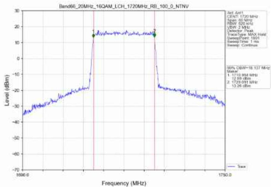
Band66_20MHz_16QAM_LCH_1720MHz_RB_100_0_NTNV
