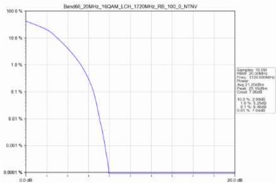
Band66_20MHz_16QAM_LCH_1720MHz_RB_100_0_NTNV
