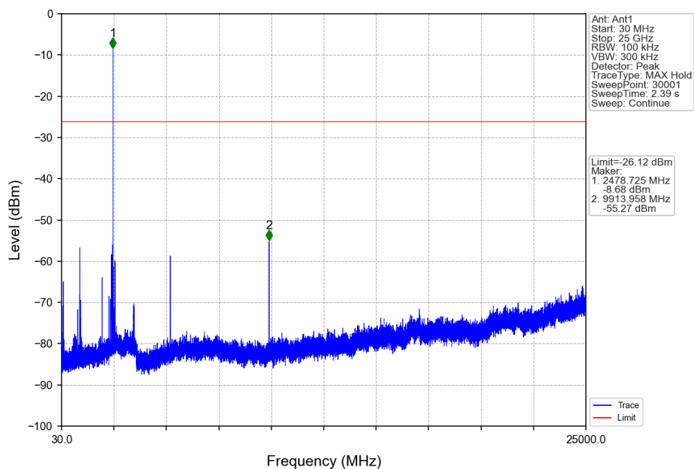
GFSK_HCH_2480MHz_Ant1_NTNV
