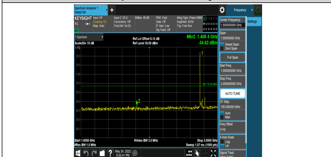
Band2-20MHz-QPSK-18900-1RB#0-Range4:1000~2000MHz
