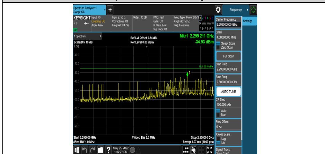
Band40-5MHz-QPSK-38750-1RB#0-Range7:2296~2300MHz
