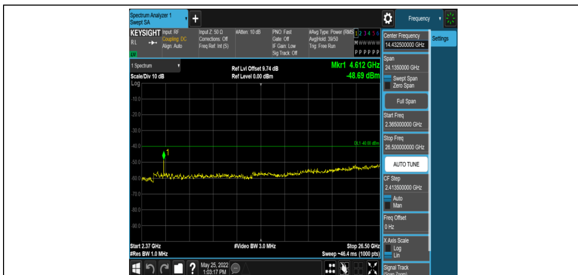
Band40-5MHz-QPSK-38725-1RB#0-Range15:2365~26500MHz
