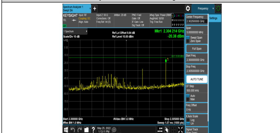
Band40-5MHz-QPSK-38775-1RB#0-Range8:2300~2305MHz
