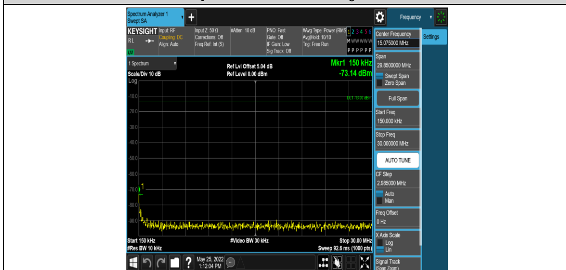
Band40-5MHz-QPSK-38775-1RB#0-Range2:0.15~30MHz
