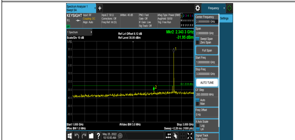
Band41-20MHz-QPSK-41490-1RB#0-Range4:1000~3000MHz
