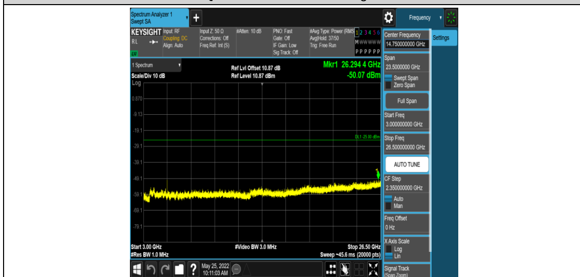
Band41-20MHz-QPSK-41490-1RB#0-Range5:3000~26500MHz
