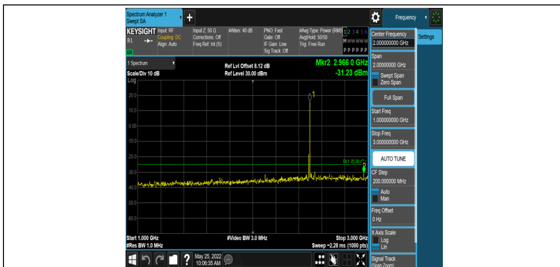
Band41-20MHz-QPSK-39750-1RB#0-Range4:1000~3000MHz
