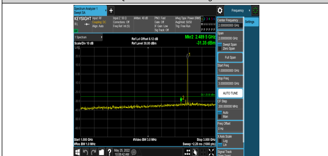
Band41-20MHz-QPSK-40620-1RB#0-Range4:1000~3000MHz
