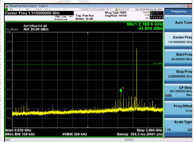
30MHz-3GHz
