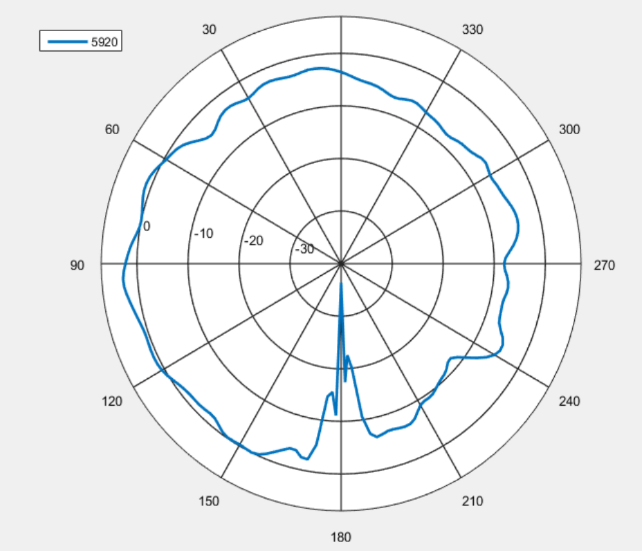
5920MHz
