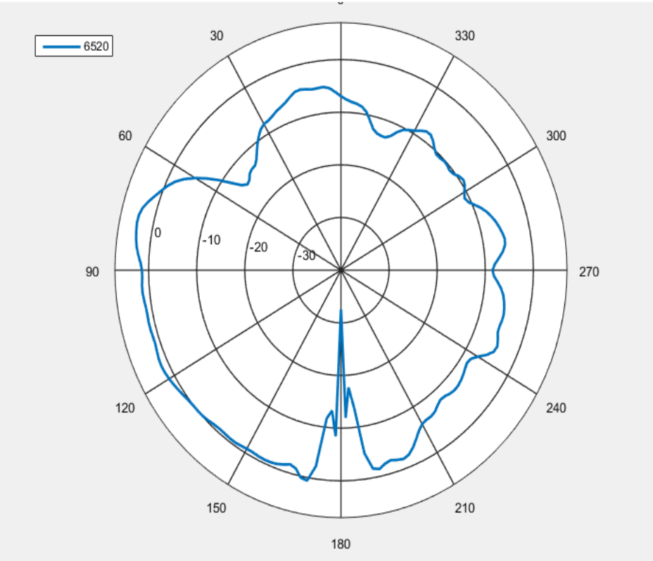
6520MHz
