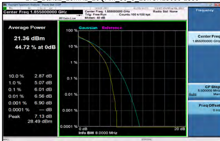
LTE Band2 10MHz 16QAM 50 0 LowCH18650-1855
