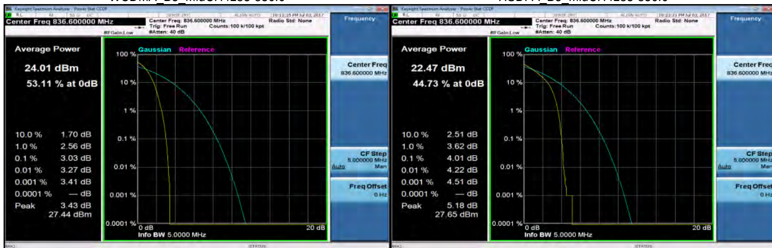
WCDMA B5 MidCH4183-836.6
