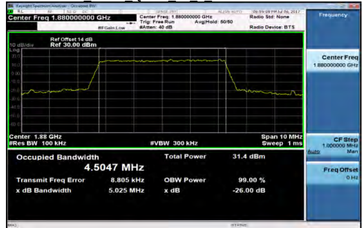
Band2 5MHz QPSK 25 0 MidCH18900-1880
