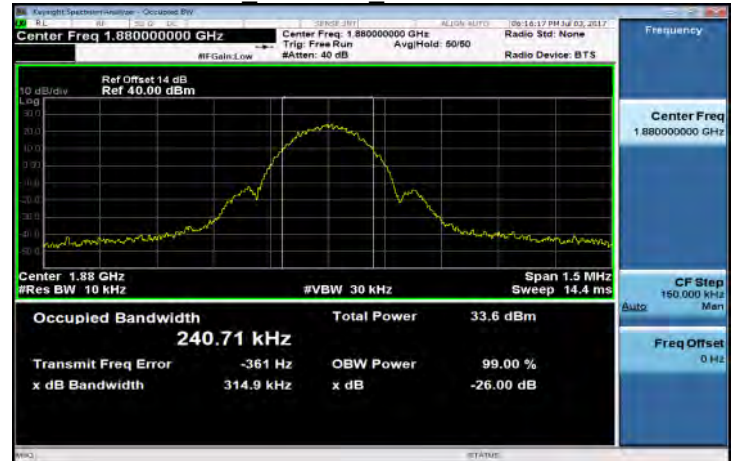
EDGE 1900MHz MidCH661-1880
