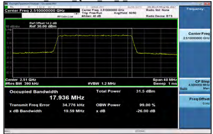
Band7 20MHz QPSK 100 0 LowCH20850-2510
