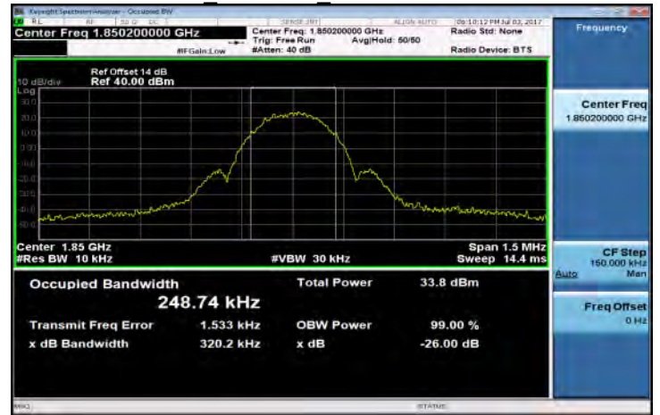
EDGE 1900MHz LowCH512-1850.2
