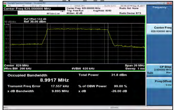
Band5 10MHz QPSK 50 0 LowCH20450-829
