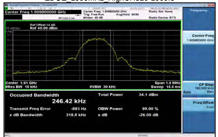
EDGE 1900MHz HighCH810-1909.8
