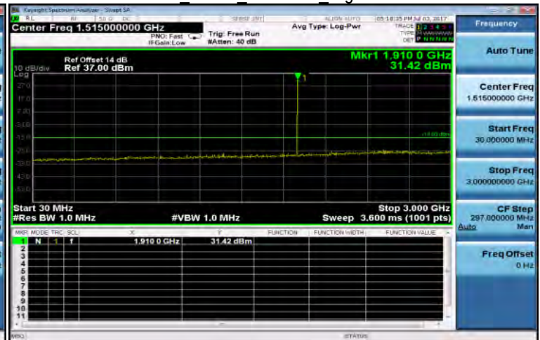
30MHz~3GHz GPRS 1900MHz HighCH810-1909.8
