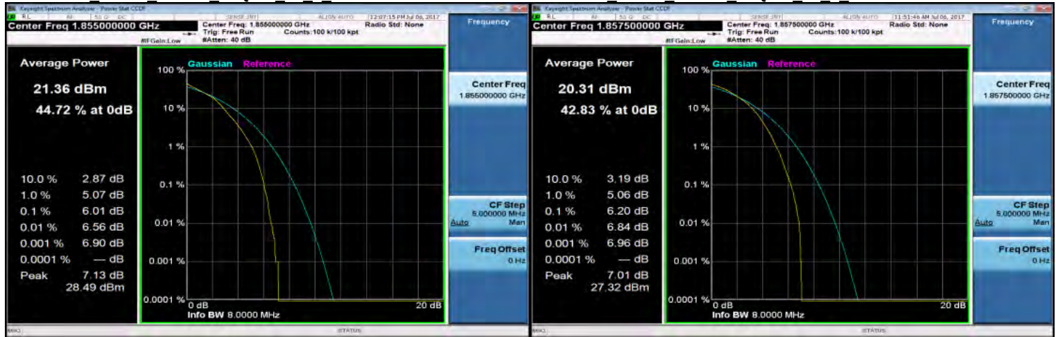
LTE Band2 10MHz 16QAM 50 0 LowCH18650-1855
