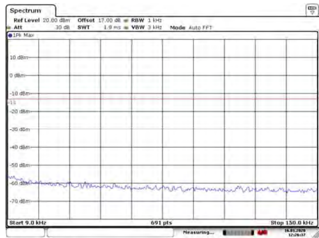
GSM 1900 CH- Middle 9kHz ~ 150kHz
