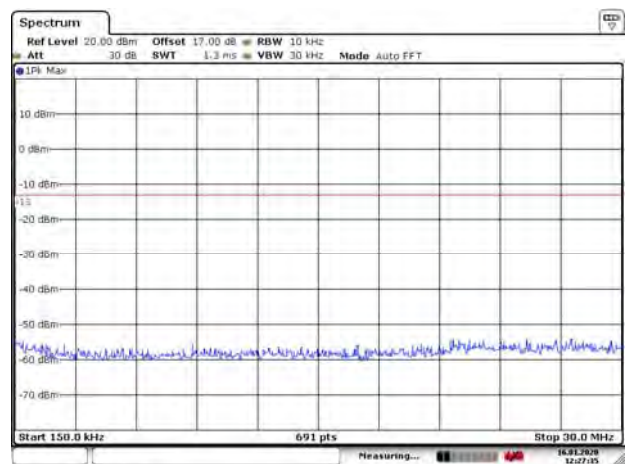
GSM 1900 CH- Middle 150kHz ~ 30MHz
