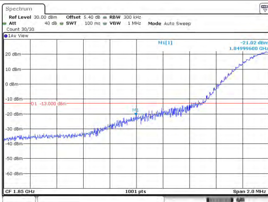
Band2-20MHz-64QAM-18700-1RB#0
