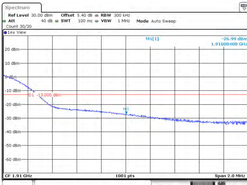
Band2-20MHz-16QAM-19100-100RB#0
