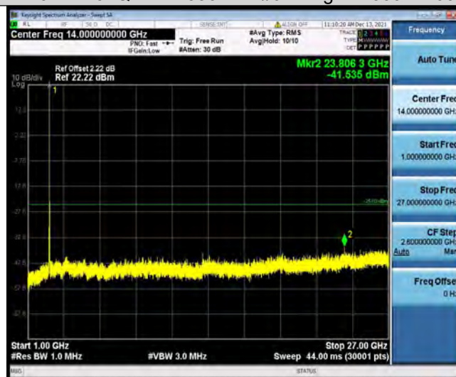
Band7-20MHz-64QAM-21350-1RB#0-Range2:1000~27000MHz
