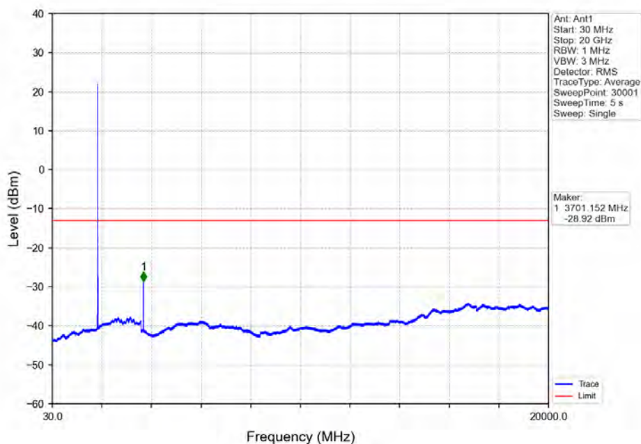
Band2_10MHz_16QAM_LCH_1855MHz_RB_50_0_NTNV
