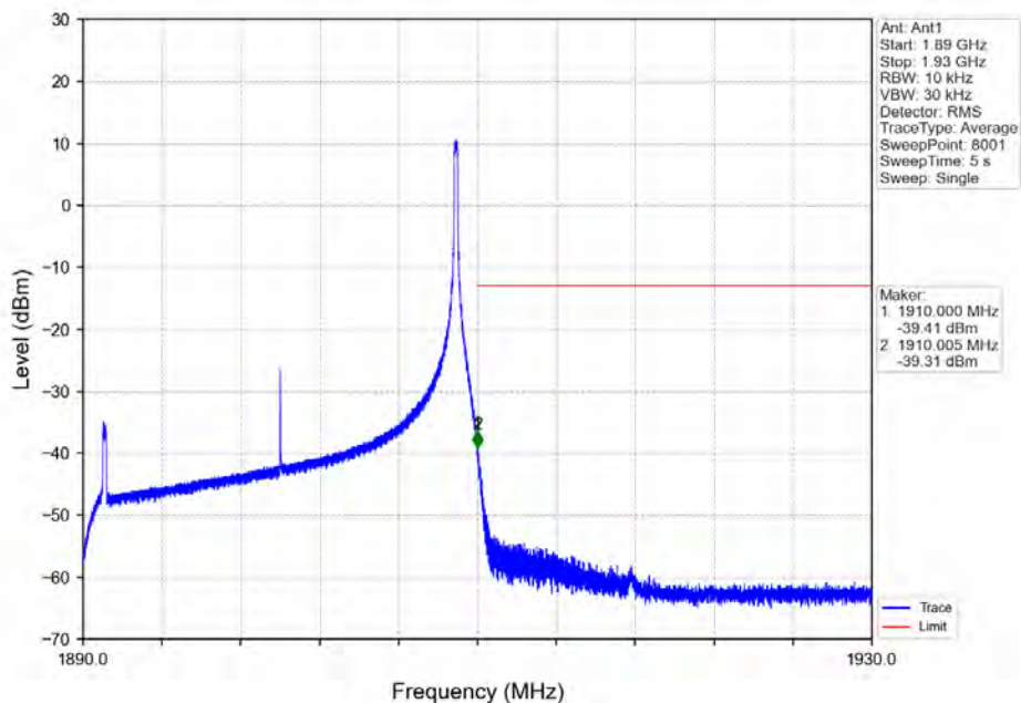
Band2_20MHz_64QAM_HCH_1900MHz_RB_1_99_NTNV
