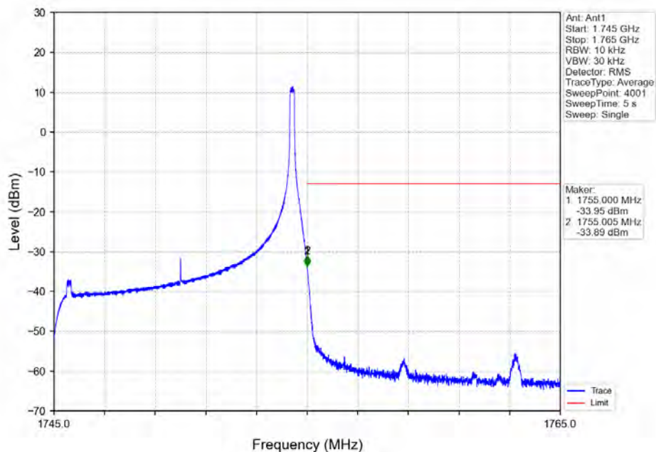
Band4_10MHz_QPSK_HCH_1750MHz_RB_1_49_NTNV
