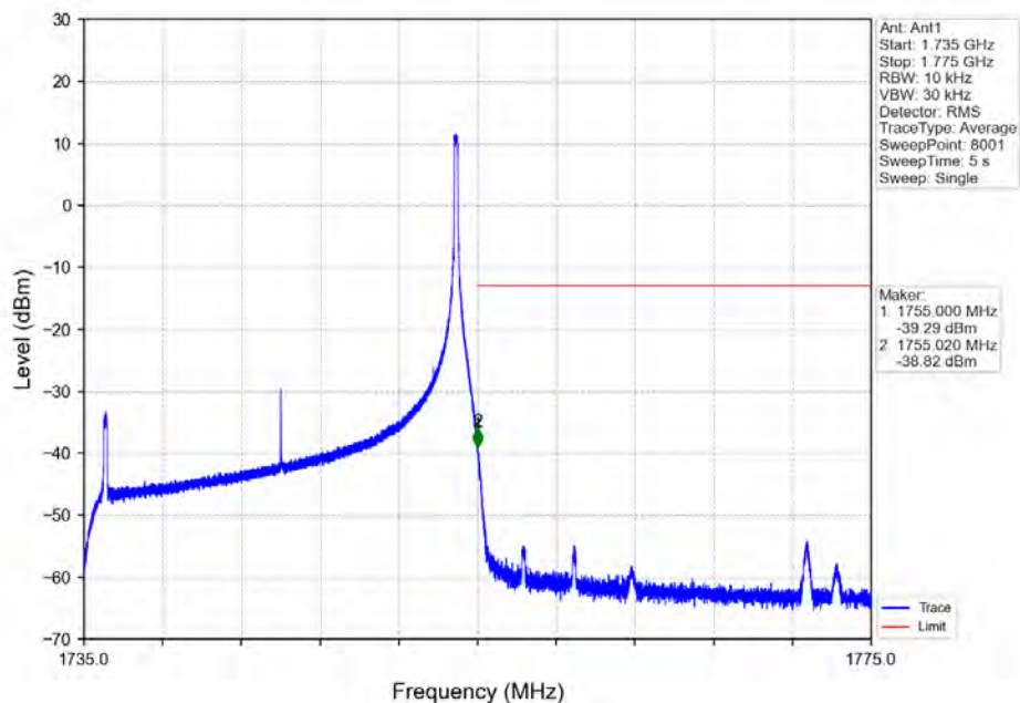
Band4_20MHz_QPSK_HCH_1745MHz_RB_1_99_NTNV
