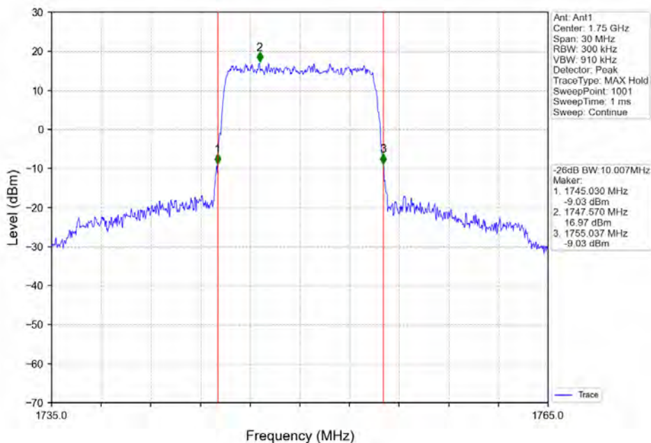
Band4 10MHz QPSK HCH 1750MHz RB 50 0 NTNV
