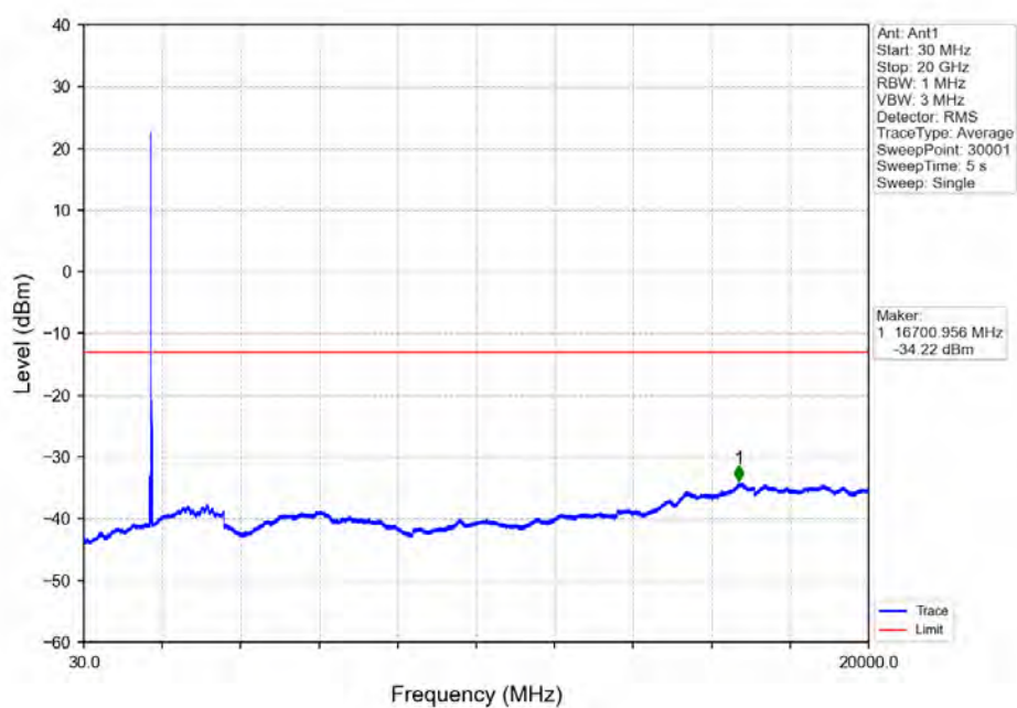
Band4_20MHz_QPSK_HCH_1745MHz_RB_1_99_NTNV
