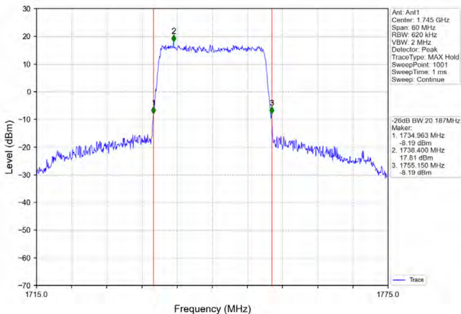
Band4_20MHz_QPSK_HCH_1745MHz_RB_100_0_NTNV
