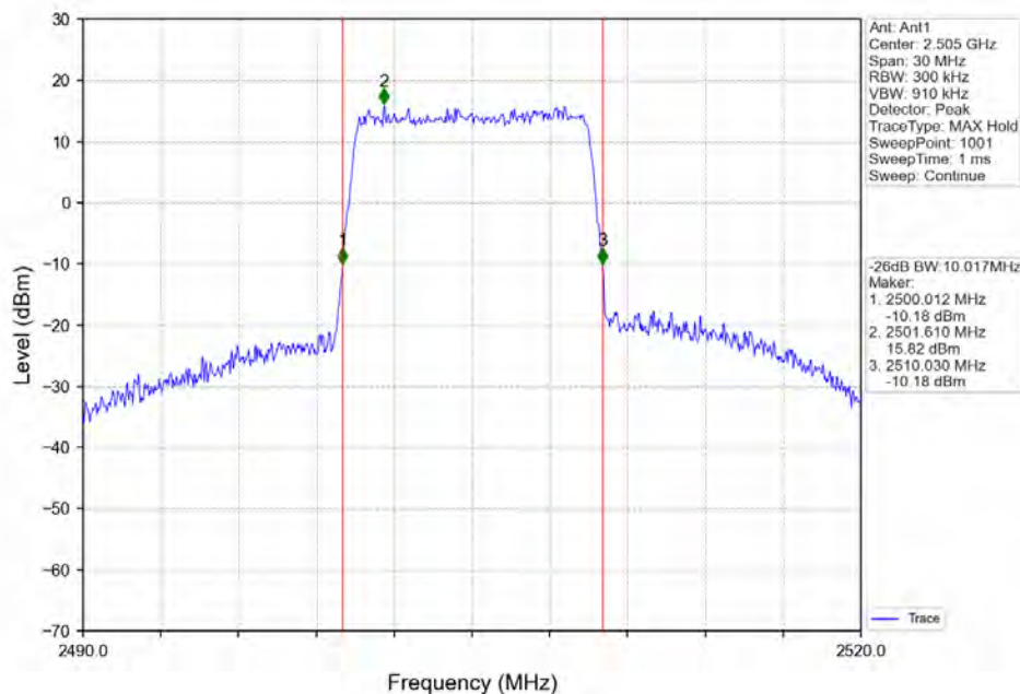
Band7_10MHz_QPSK_LCH_2505MHz_RB_50_0_NTNV
