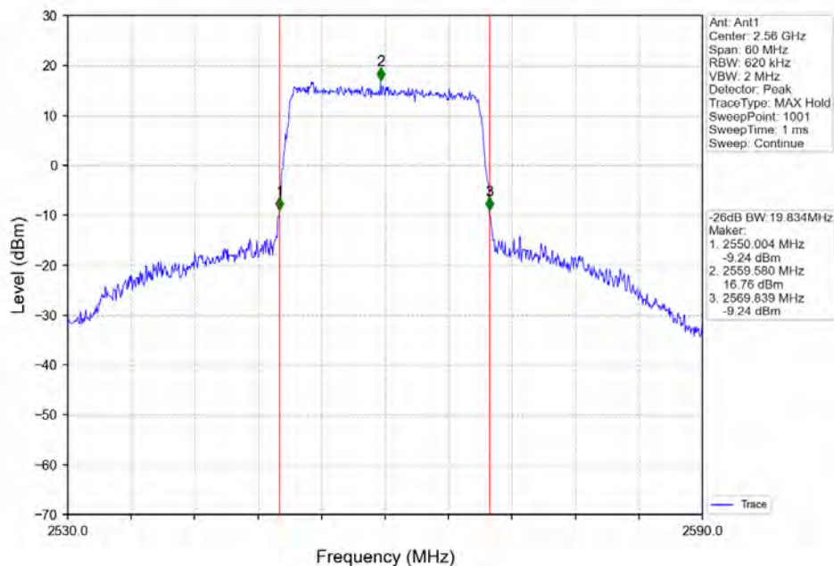
Band7 20MHz QPSK HCH 2560MHz RB 100 0 NTVN
