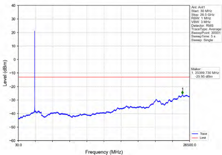
Band7_20MHz_QPSK_HCH_2560MHz_RB_1_99_NTNV
