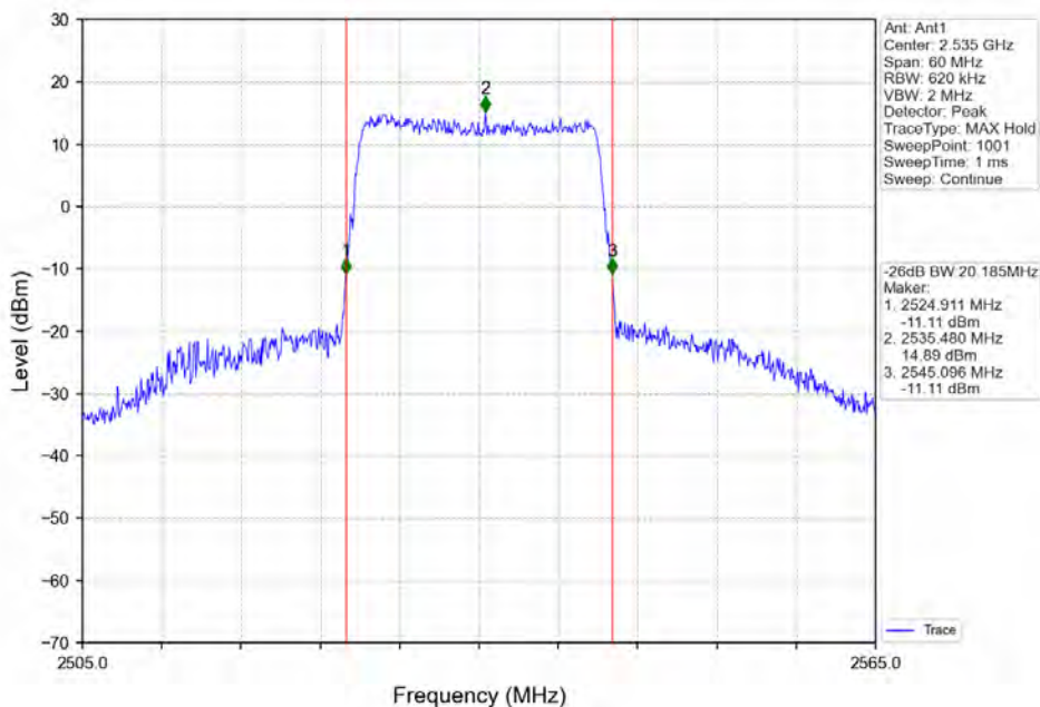
Band7 20MHz 16QAM MCH 2535MHz RB 100 0 NTNV
