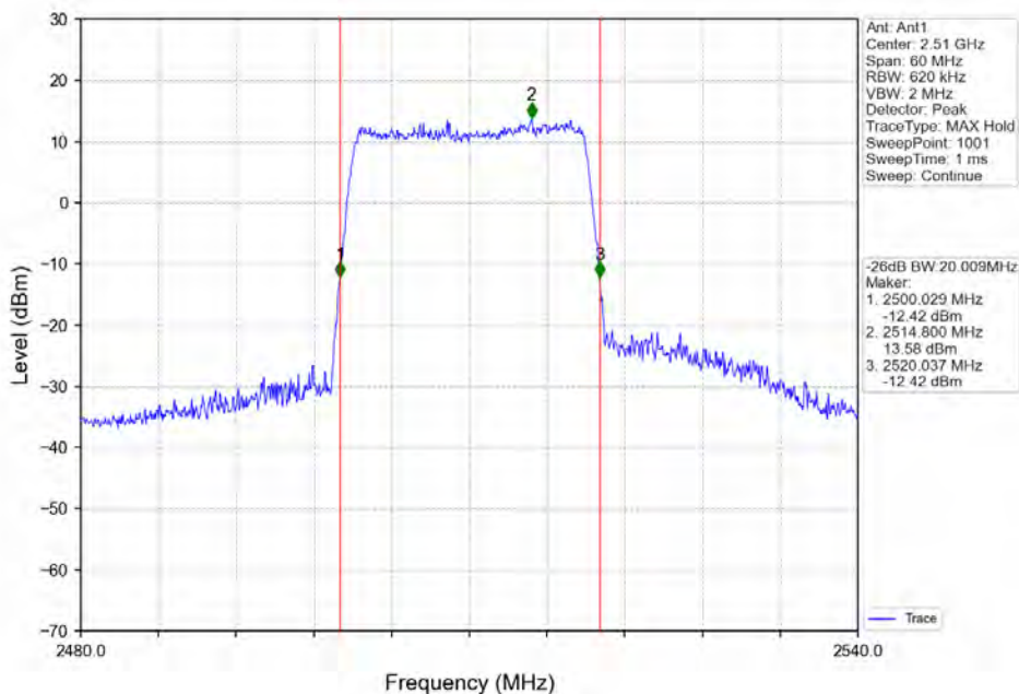
Band7 20MHz 64QAM LCH 2510MHz RB 100 0 NTNV
