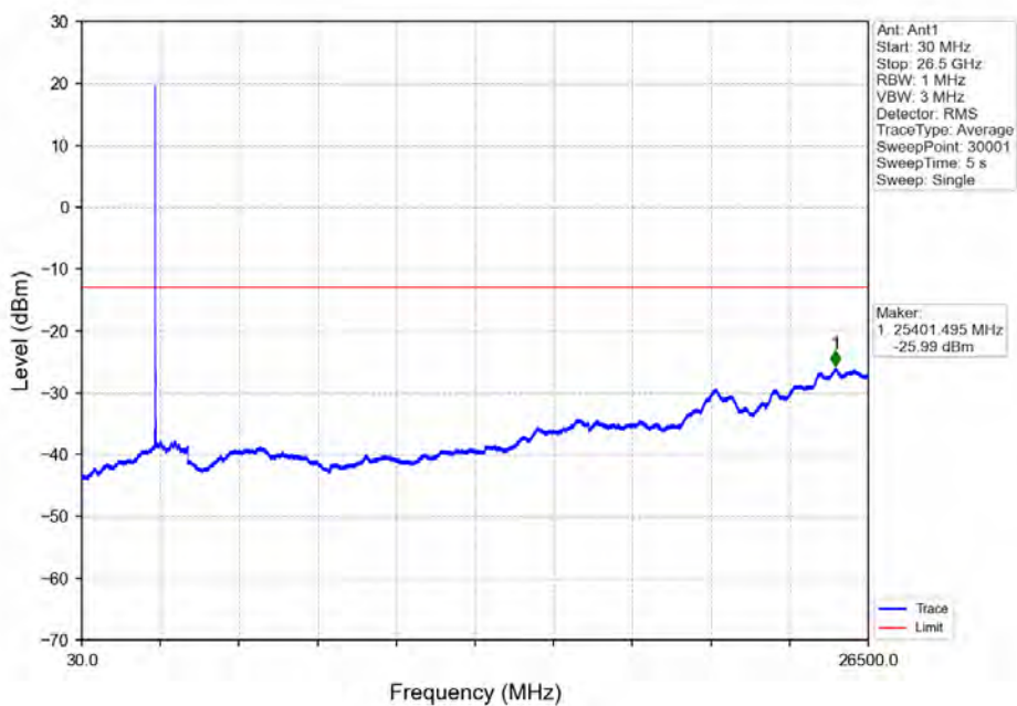
Band7 15MHz 16QAM LCH 2507.5MHz RB 75 0 NTNV
