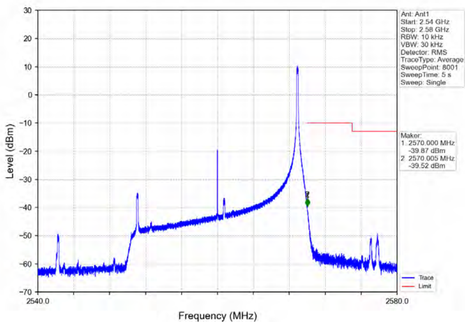
Band7 20MHz 16QAM HCH 2560MHz RB 100 0 NTNV
