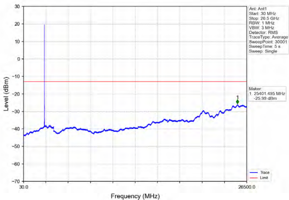
Band7 15MHz 16QAM LCH 2507.5MHz RB 75 0 NTV
