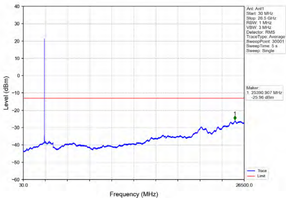
Band7 10MHz QPSK HCH 2565MHz RB 1 49 NTV
