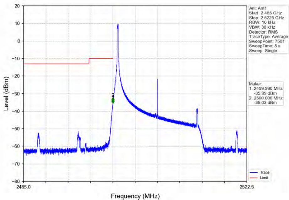
Band7 15MHz 16QAM LCH 2507.5MHz RB 1 0 NTV
