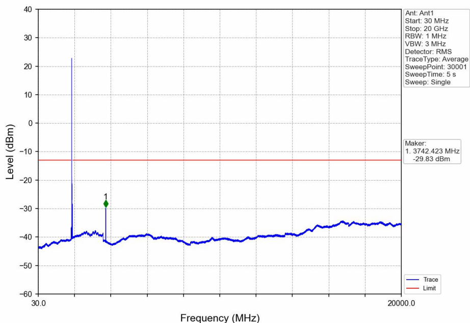
Band2_20MHz_QPSK_MCH_1880MHz_RB_1_0_NTNV
