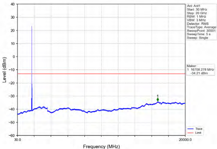
Band66_20MHz_QPSK_MCH_1745MHz_RB_1_0_NTNV
