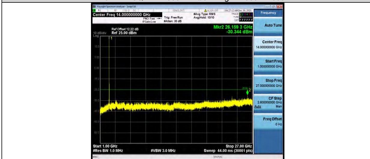
Band7-20MHz-16QAM-21350-1RB#0-Range2:1000~27000MHz
