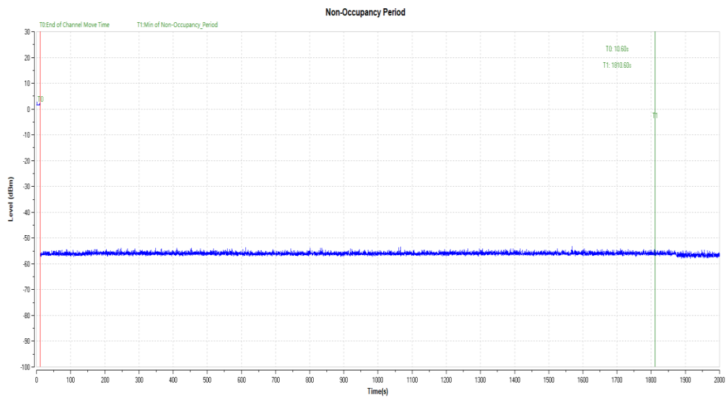
11AC80SISO_5290
