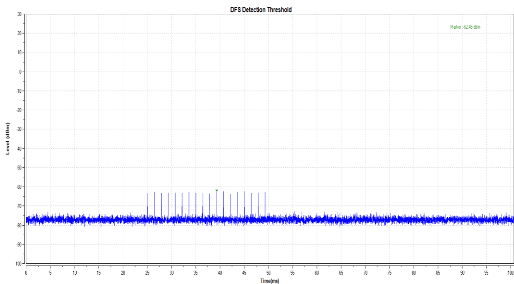
11AC80SISO_5290_Type0
