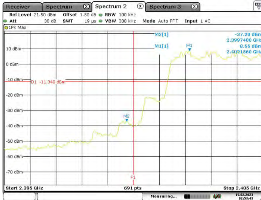
2DH5_Ant1_Low_Hop_2402
