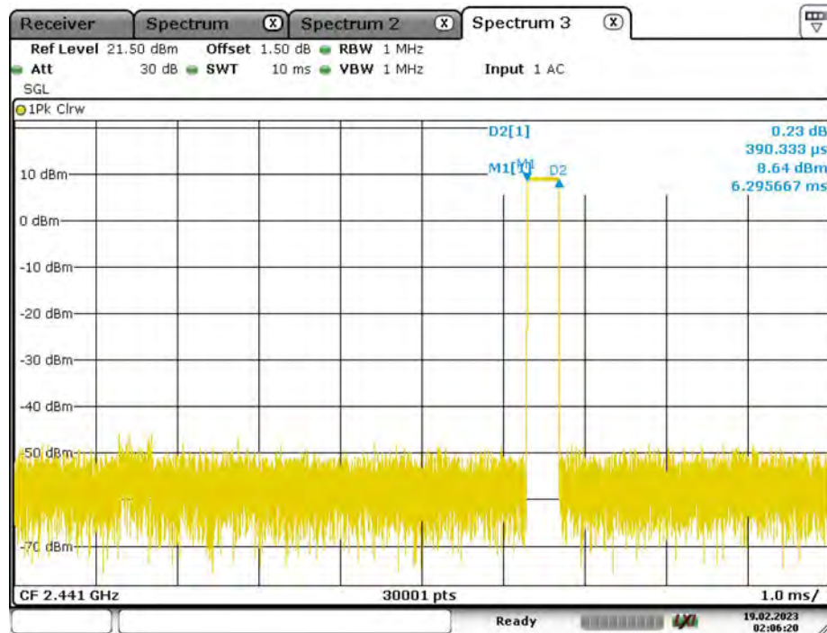
DH1_Ant1_Hop
