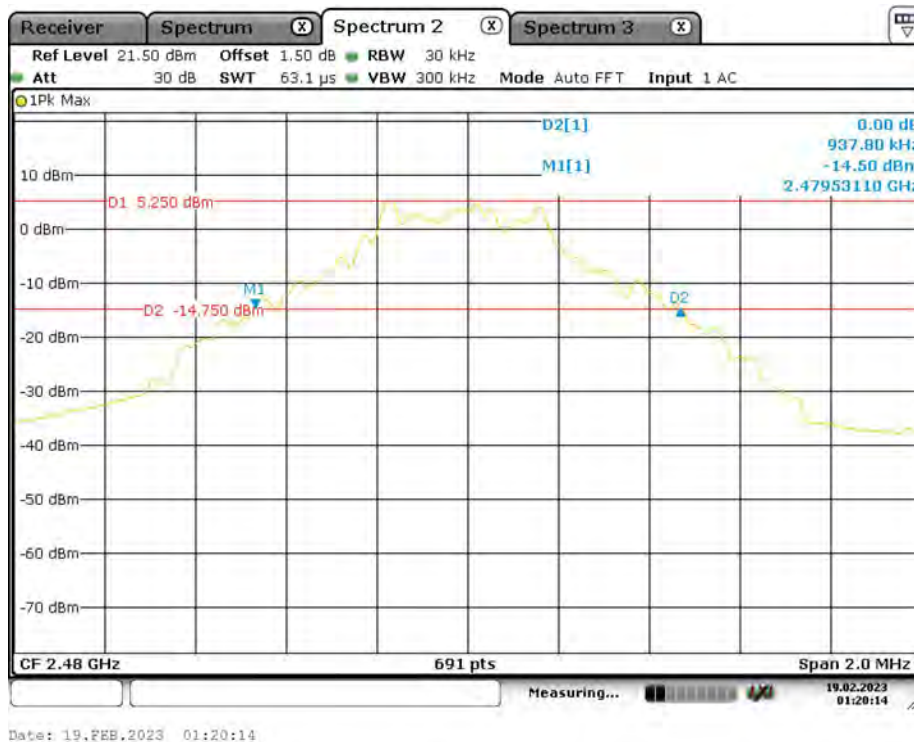
DH5_Ant1_2480
