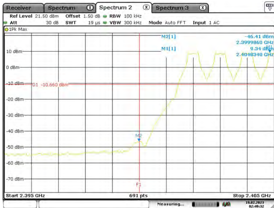
DH5_Ant1_Low_Hop_2402
