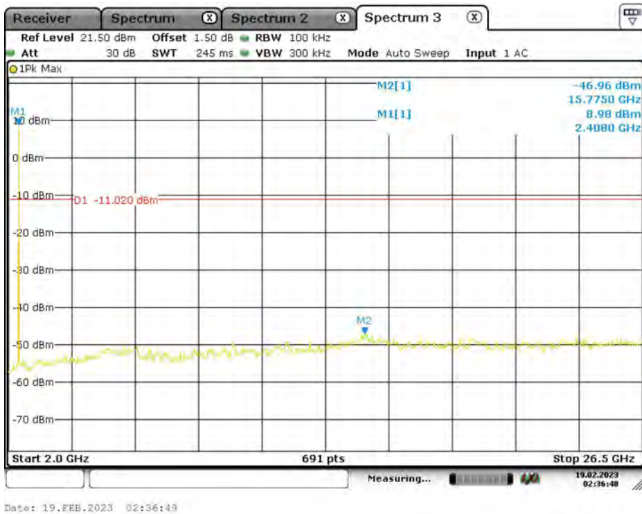
DH5_Ant1_2402_2000~26500
