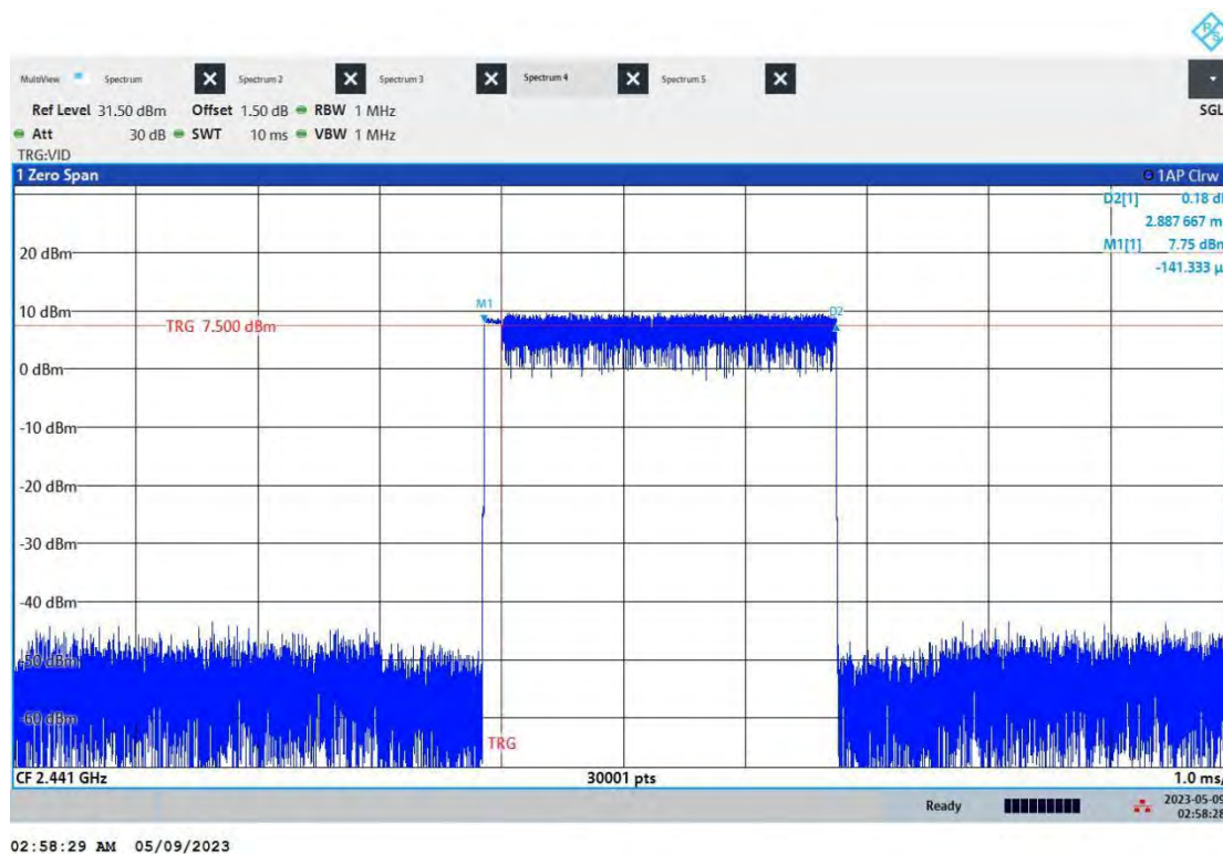
2DH5_Ant1_Hop
