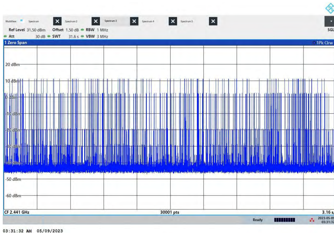
DH5_Ant1_Hop
