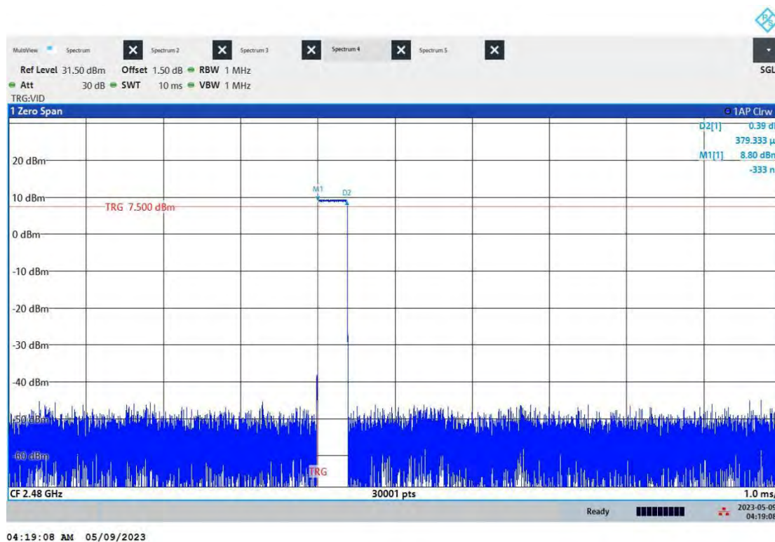
DH1_Ant1_Hop
