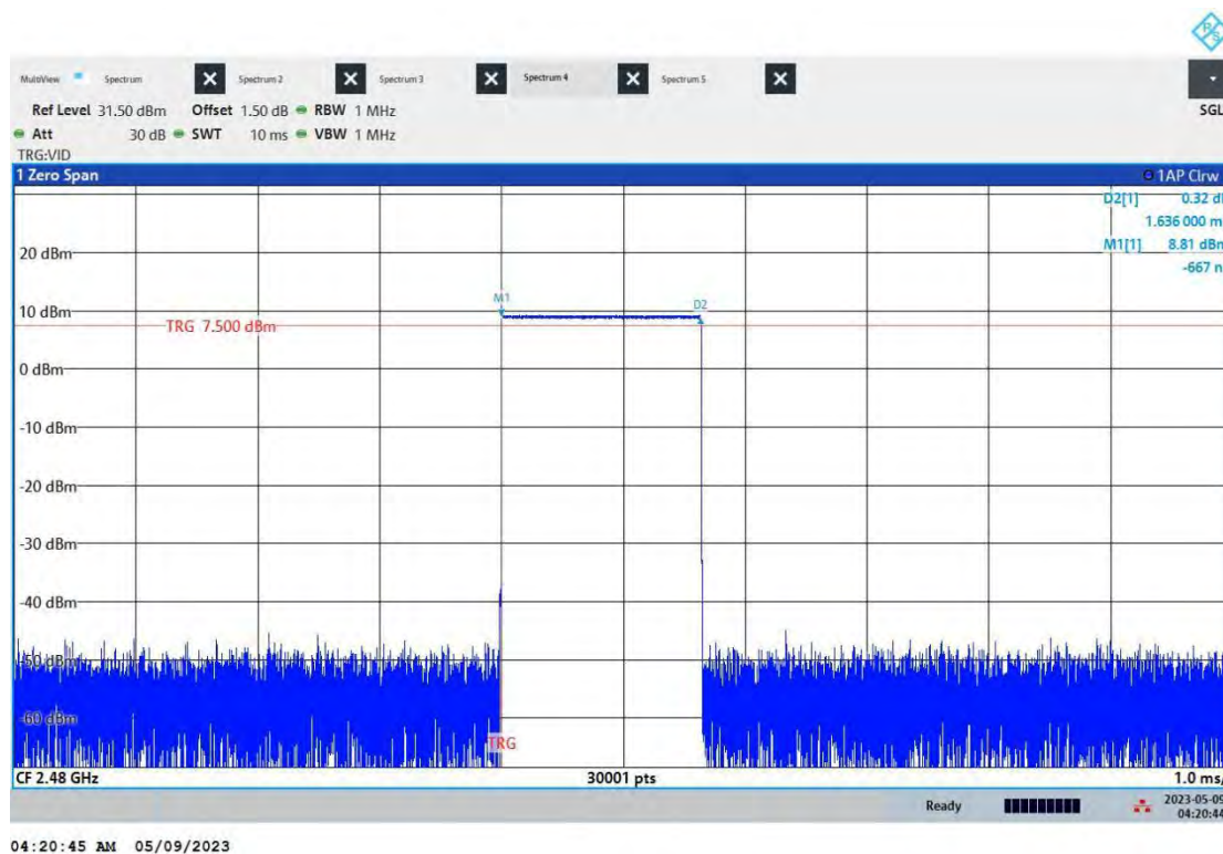
DH3_Ant1_Hop
