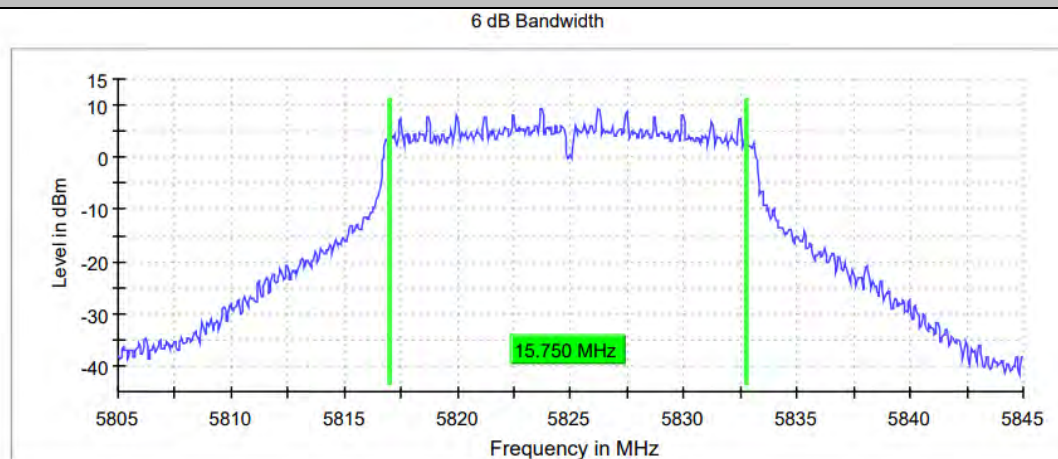
11A_Ant0_5825
