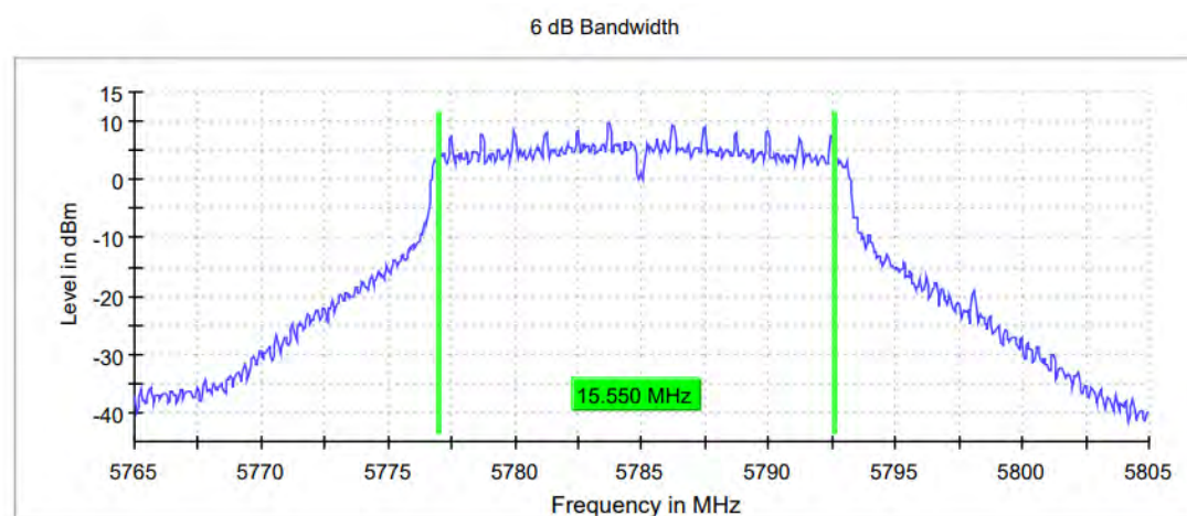
11A_Ant0_5785
