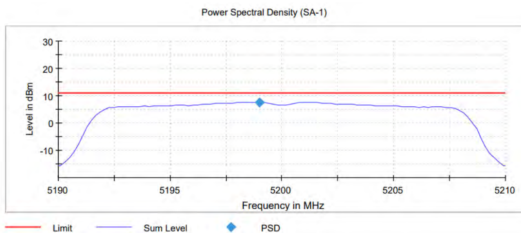
11A_An0_5200
