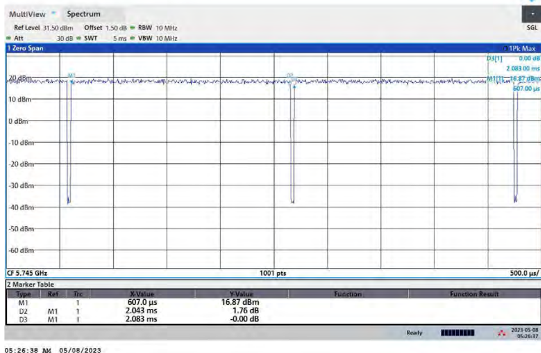
Band4-11A_Ant0_5745
