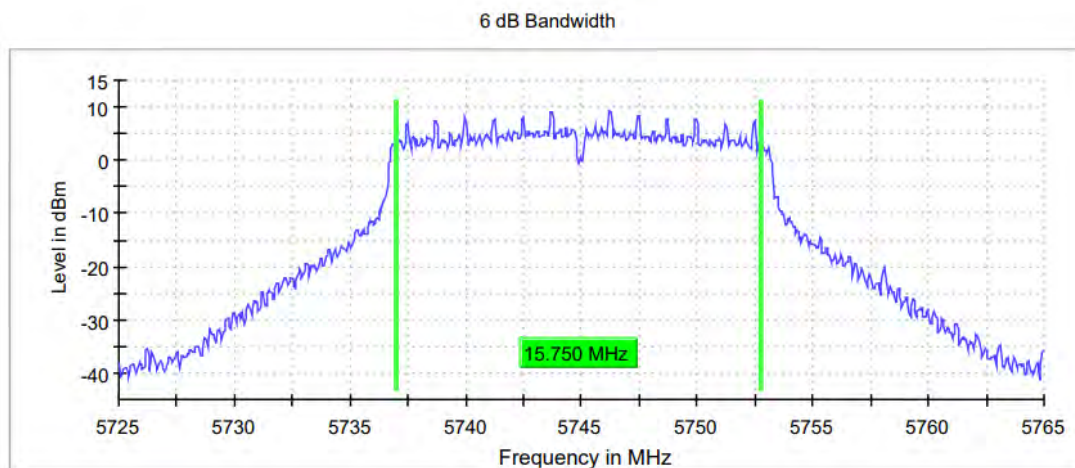
11A_Ant0_5745
