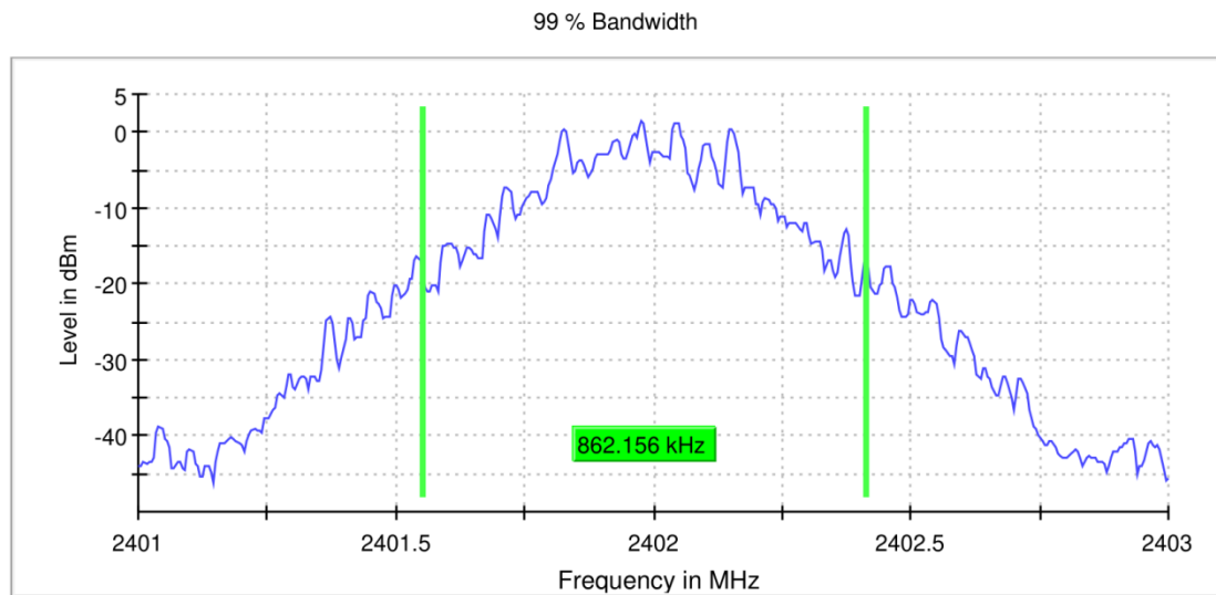
DH5_ANT0_2402
