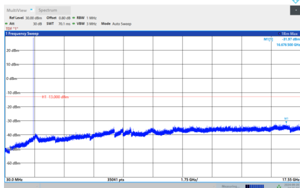
Band4-1.4MHz-QPSK-20393-1RB#0-Range:30~1755 0MHz
