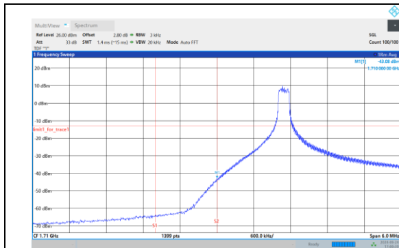
Band4-20MHz-QPSK-20300-1RB#99
