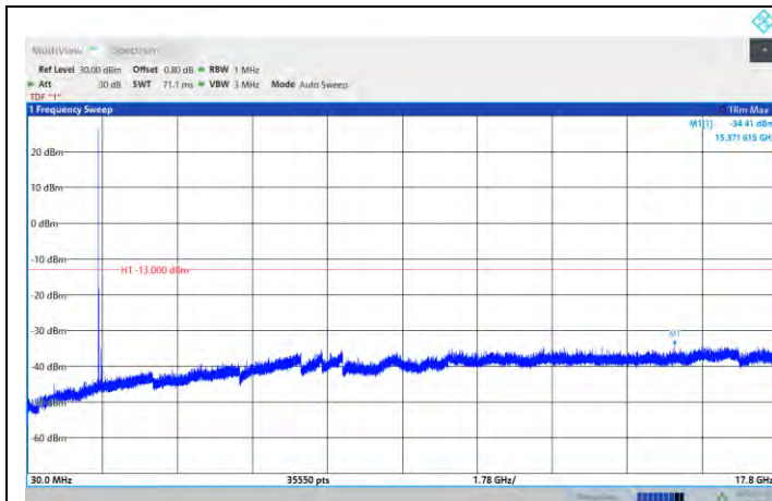
N66-PC3-5MHz-L-DFT-QPSK-Edge_1RB_Left
