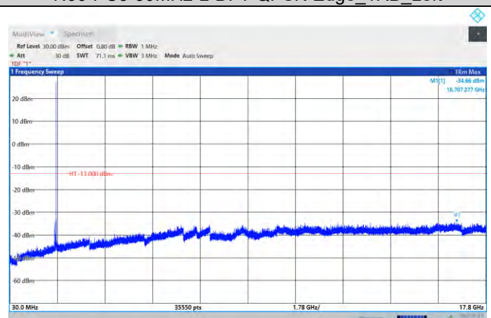
N66-PC3-30MHz-H-DFT-QPSK-Edge_1RB_Left
