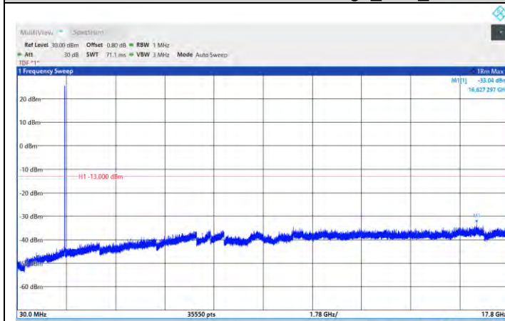
N66-PC3-10MHz-M-DFT-QPSK-Edge_1RB_Left
