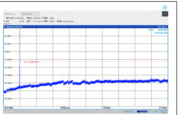
N66-PC3-5MHz-M-DFT-QPSK-Edge_1RB_Left
